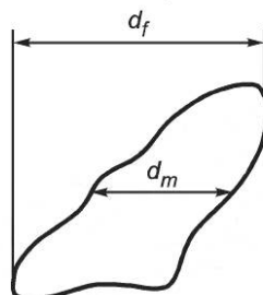
Рисунок 2 — Определение фактора формы d_f/d_m
