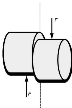
Рисунок 3 — Схема испытания
