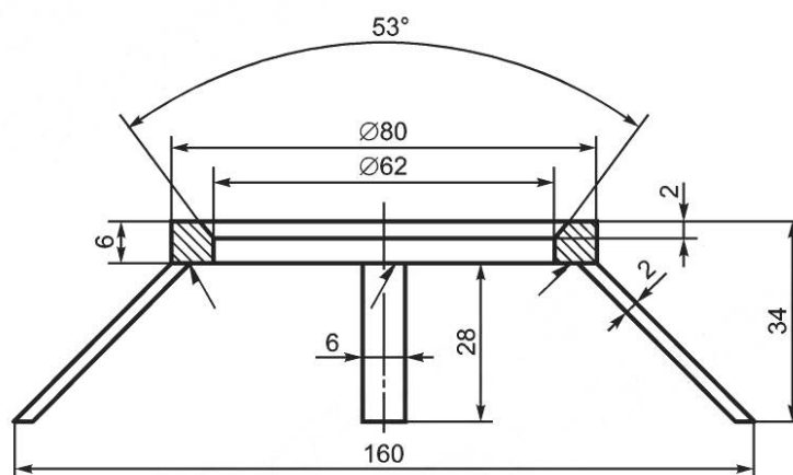
Рисунок 3 — Подставка
