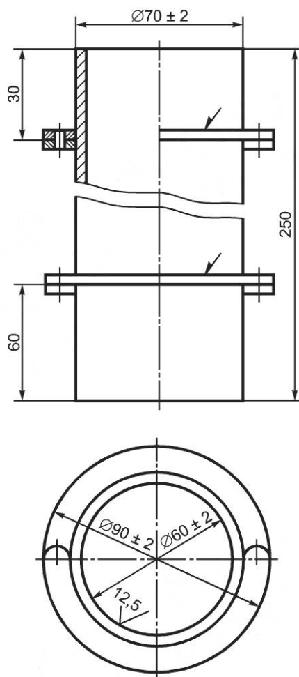
Рисунок 6 — Разъемный кожух
