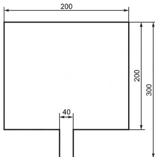
Рисунок 4 — Пластина толщиной 2—3 мм
