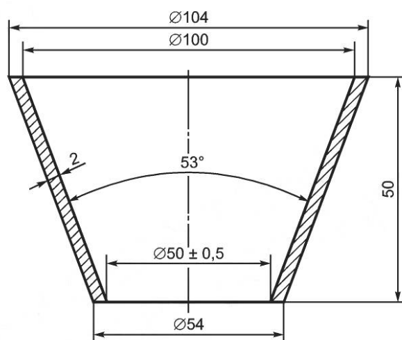
Рисунок 2 — Коническая емкость
