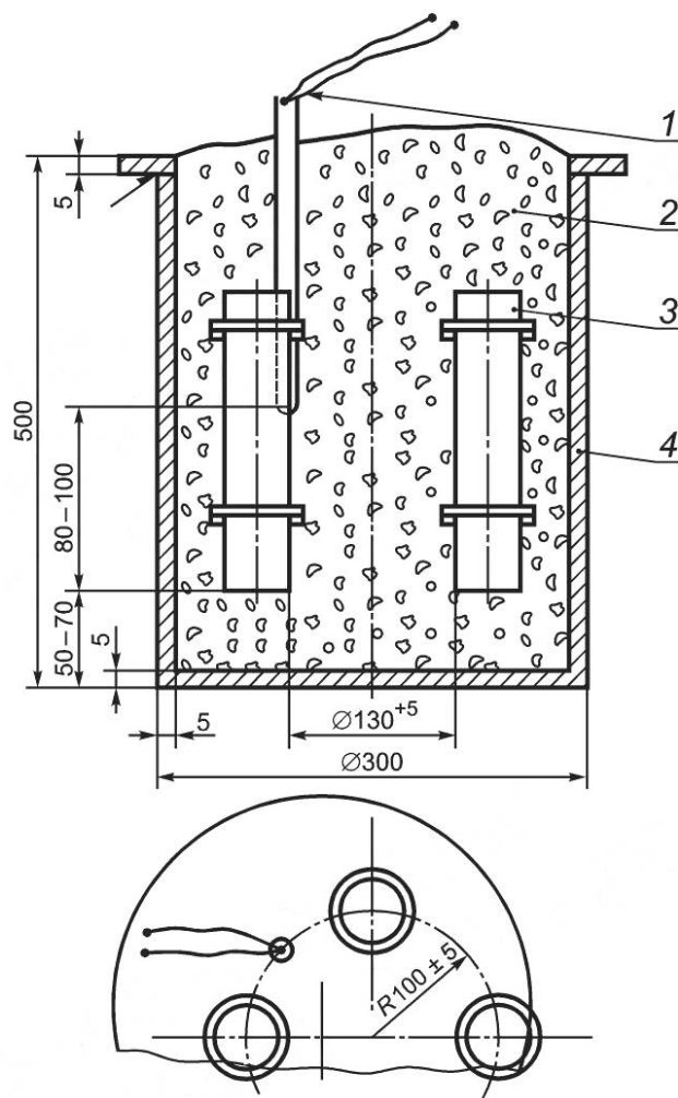
1 — хромель-алюмелевая термopapa в чехле; 2 — пересыпочный кокс; 3 — кожух с массой; 4 — контейнер
