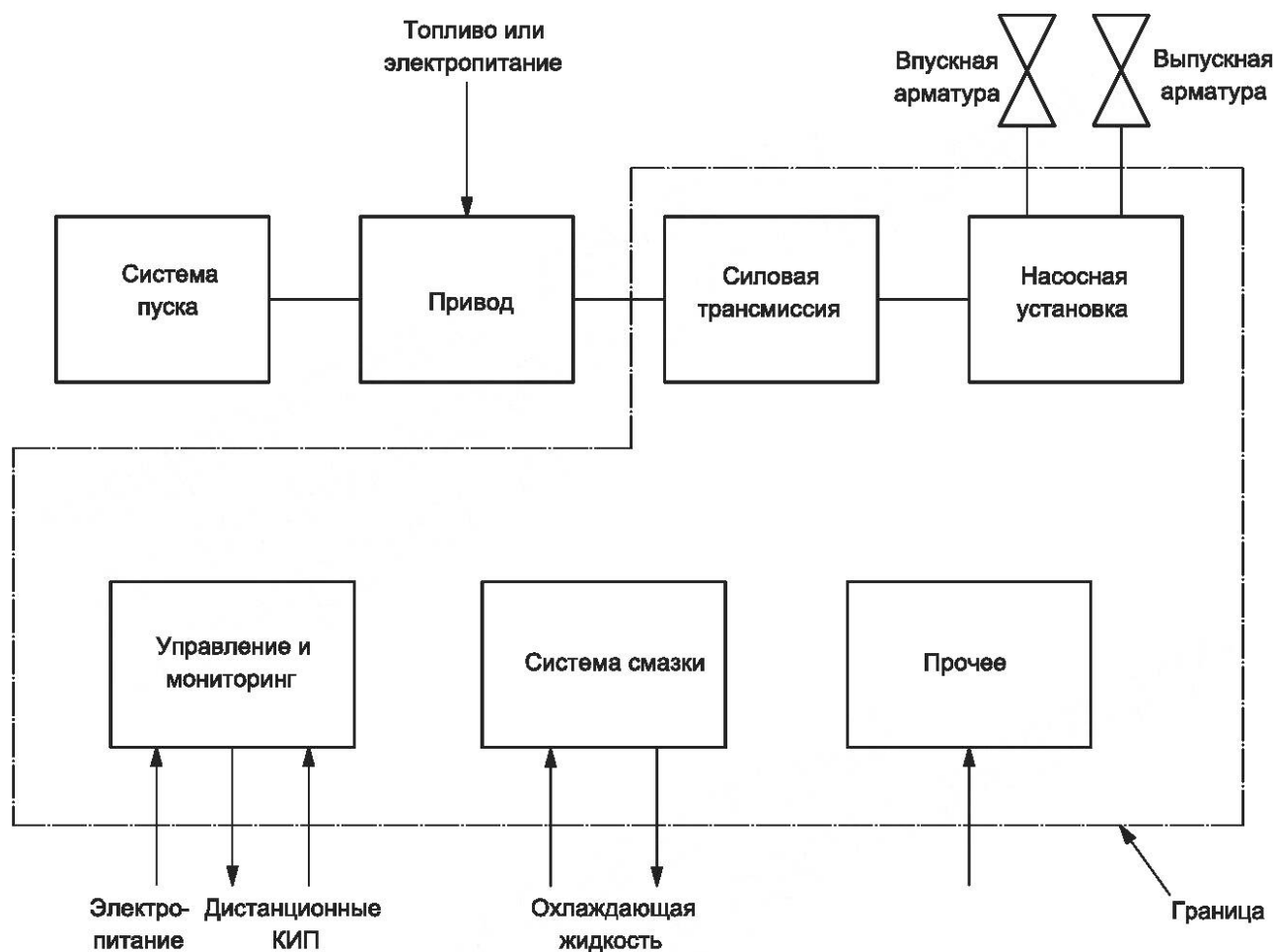
Рисунок А.7 — Определение границ. Насосы
