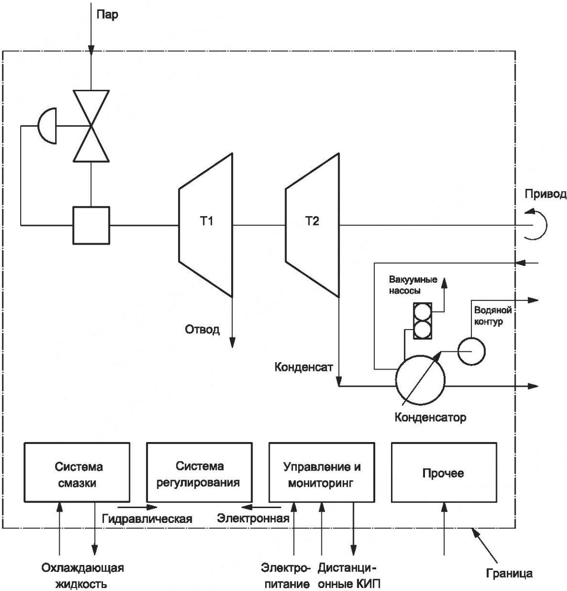
T1 — ступень турбины 1; T2 — ступень турбины 2 Рисунок А.8 — Определение границ. Паровые турбины
