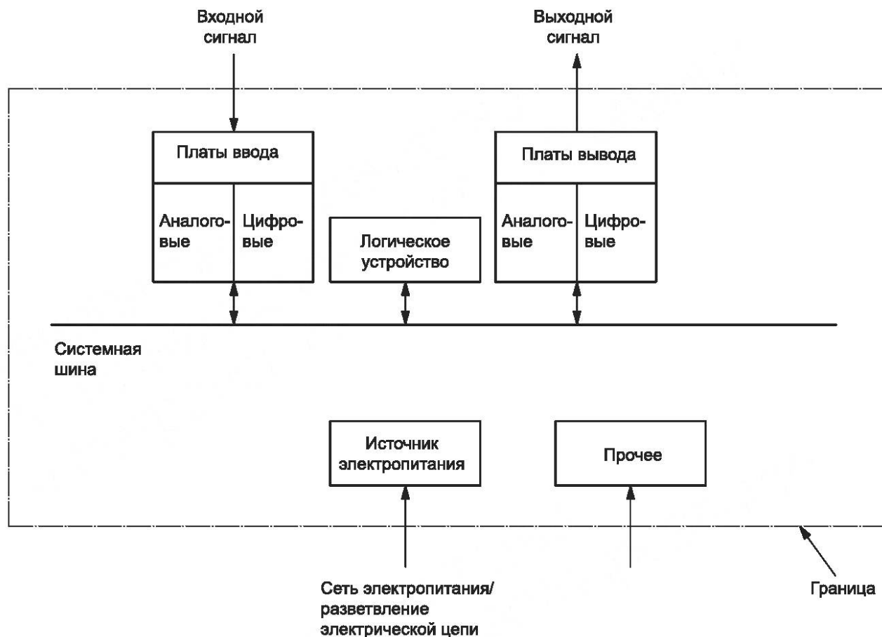
Рисунок А.26 — Определение границ. Блоки управления с логической схемой
