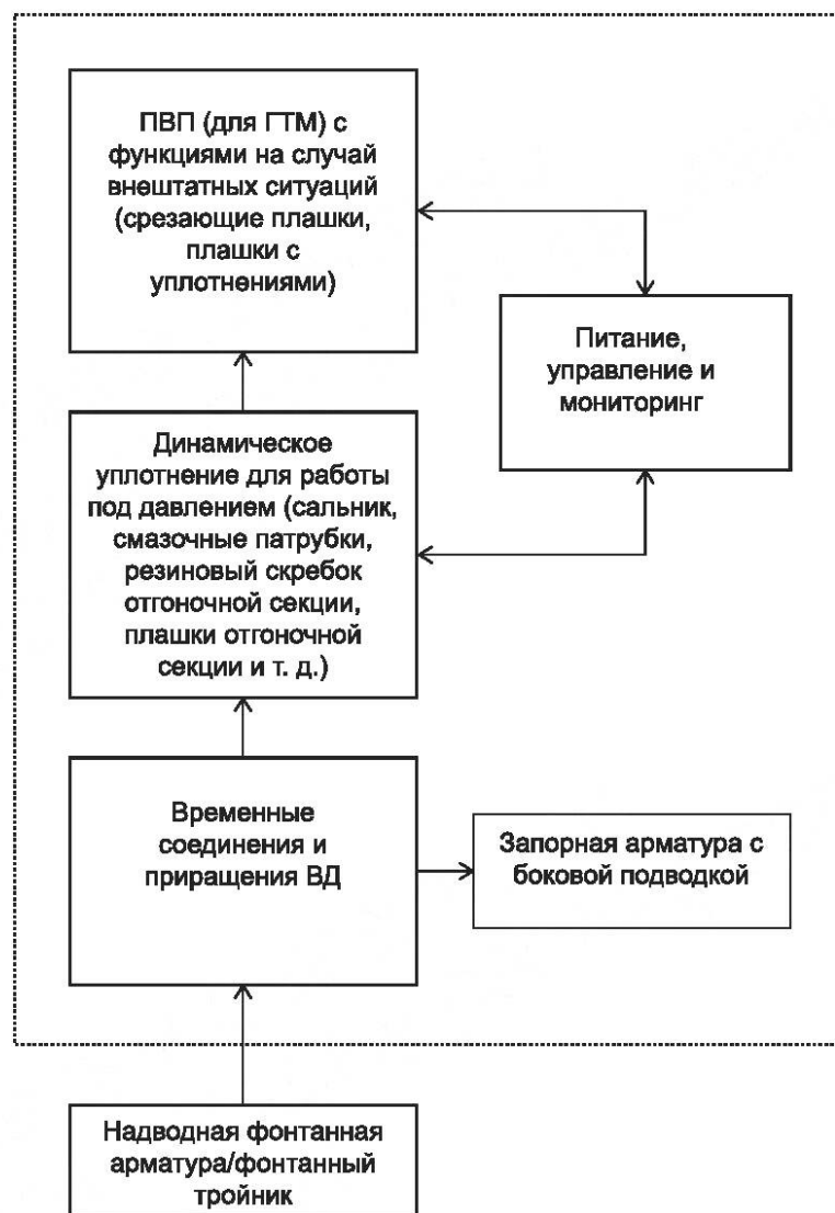
Рисунок А.42 — Определение границ. Наземное противовыбросовое оборудование (для ГТМ)
