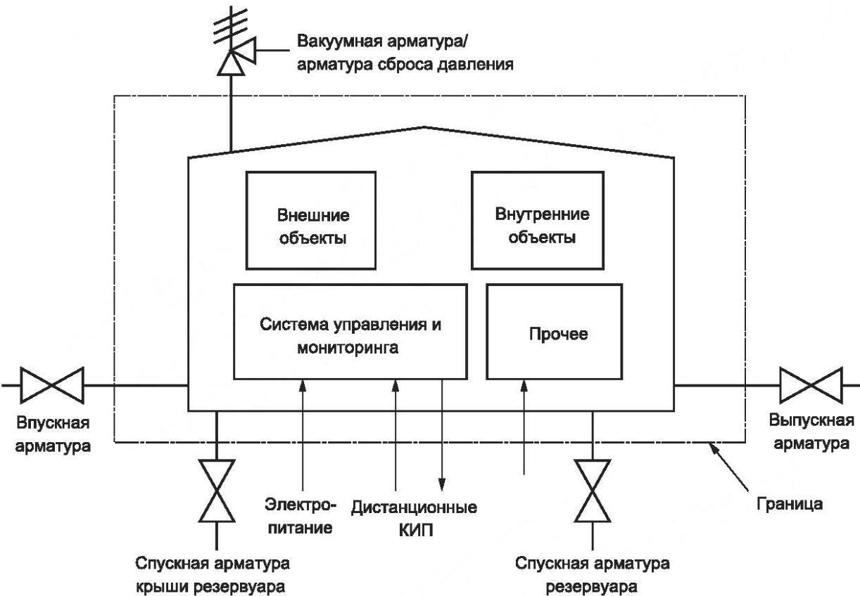
Рисунок А.18 — Определение границ. Резервуары нефтехранилища
