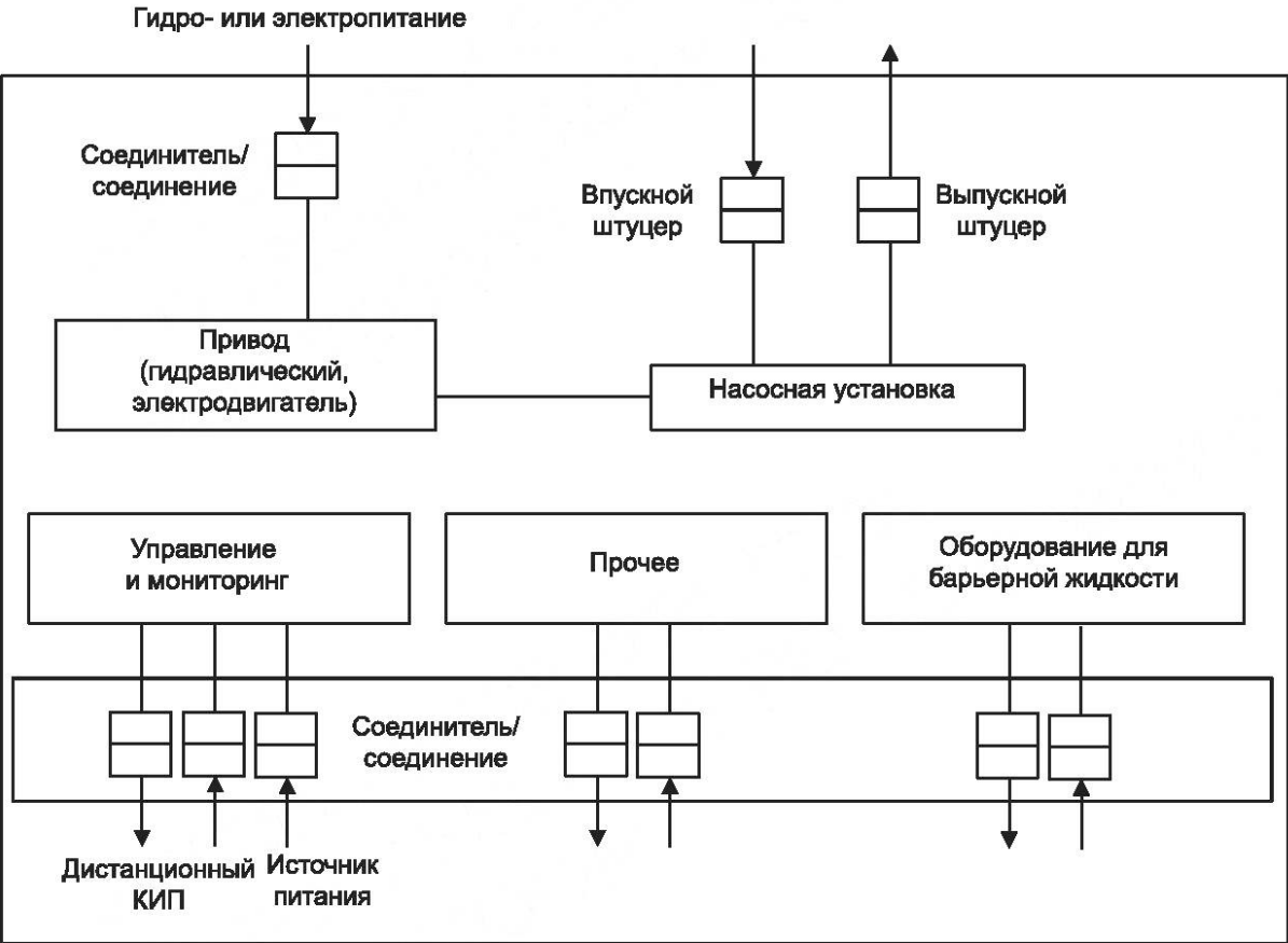
Рисунок А.33 — Определение границ. Подводные насосы
