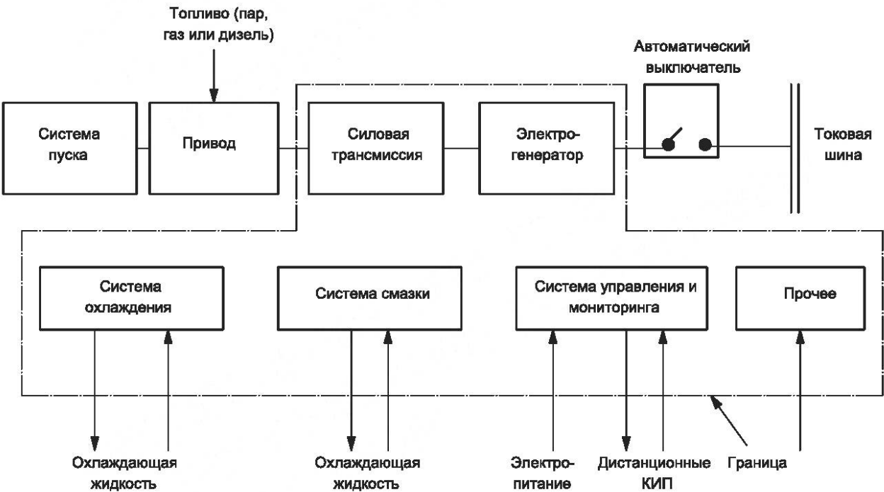
Рисунок А.4 — Определение границ. Электрогенераторы
