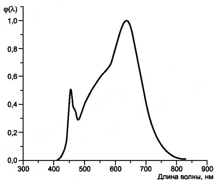
Рисунок Г.1 — Относительное спектральное распределение энергии излучения светодиодного модуля теплого белого света с коррелированной цветовой температурой 3050 К
