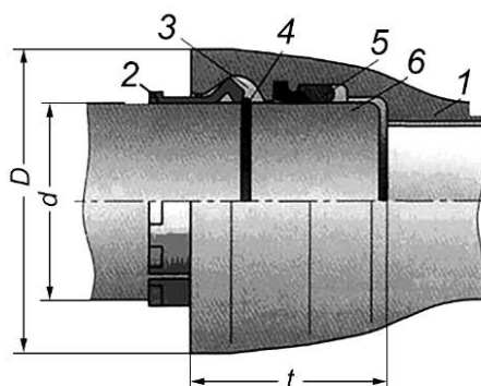
D, d — наружные диаметры раструба и трубы; t — глубина раструба; 1 — раструб; 2 — сегмент; 3 — желобок; 4 — стопор; 5 — РУМ; 6 — гладкий конец с фаской
