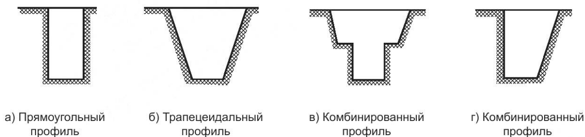
Рисунок 9.1 — Профили траншей
