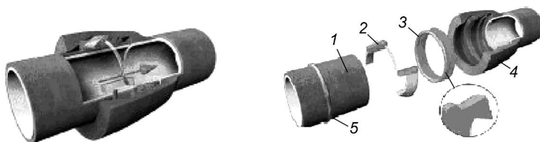
а) Общий вид в сборе
