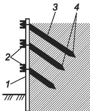
1 — шпунтовая стенка; 2 — балки; 3 — тяги; 4 — анкеры
