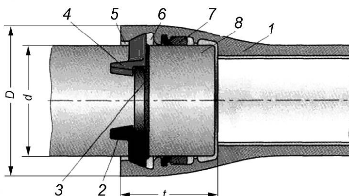
D , d — наружные диаметры раструба и трубы; t — глубина раструба; 1 — раструб; 2 — правый клин «BLS»; 3 — наварной бурт; 4 — левый клин «BLS»; 5 — сдерживающая плата; 6 — камера; 7 — РУМ; 8 — гладкий конец с фаской
