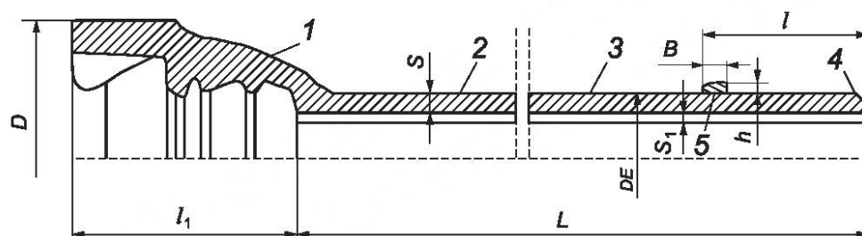
1 — раструб; 2 — тело; 3 — ЦПП; 4 — фаска; 5 — наплавленный концевой пояс
