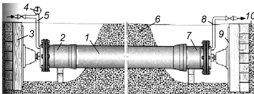
1 — ПВ и ПТНГ; 2, 7 — фасонные соединительные детали «раструб — фланец» и «гладкий конец — фланец»; 3 — упор; 4 — манометр; 5, 8 — трубы с шаровыми кранами для нагнетания воды и сброса воздуха; 6 — присыпка грунта; 9 — стальная пластина; 10 — прочная грунтовая стенка
