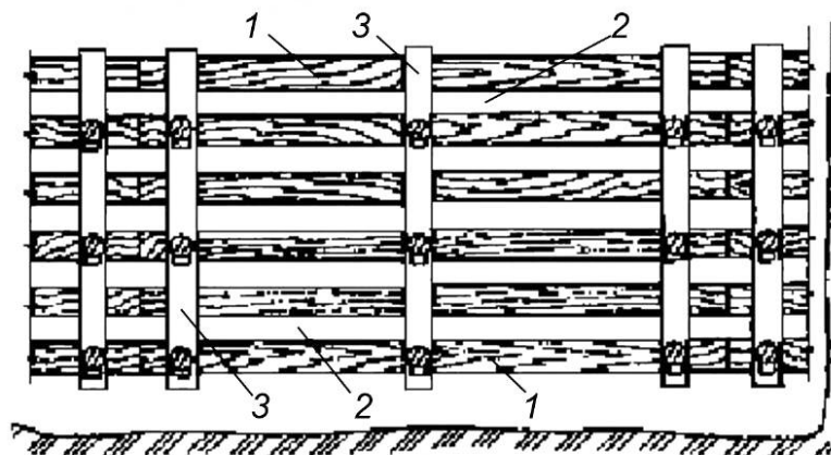
а) Вид стенки траншеи
