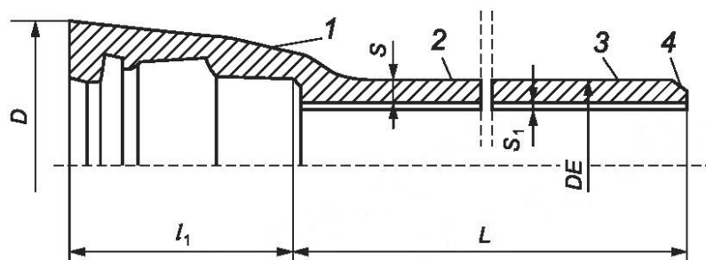
1 — раструб; 2 — тело трубы; 3 — ЦПП; 4 — фаска
