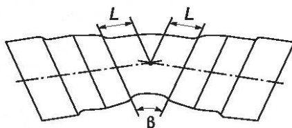
L — расстояние от точки изгиба до раструбов; \beta — угол изгиба
