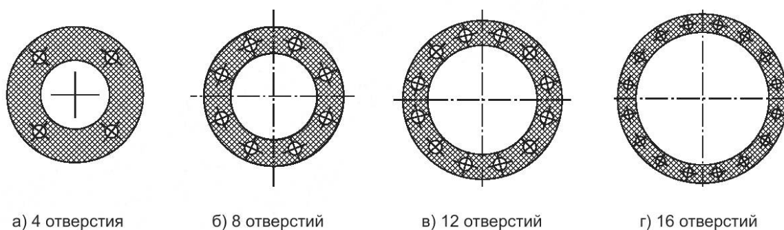
Рисунок 7.10 — Расположение отверстий в плоских прокладках для фланцевых соединений ТИ из ВЧШГ
