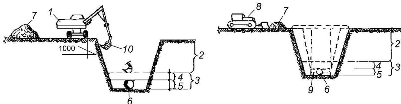
а) Засыпка экскаватором-планировщиком
