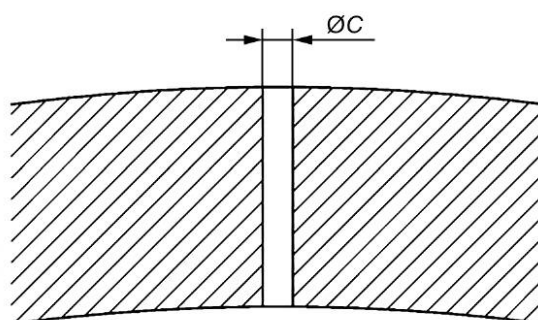
с) Сквозное сверленное отверстие
