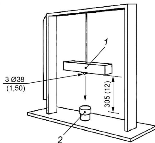
1 — стальная плита; 2 — образец; 3 — стальной прут
