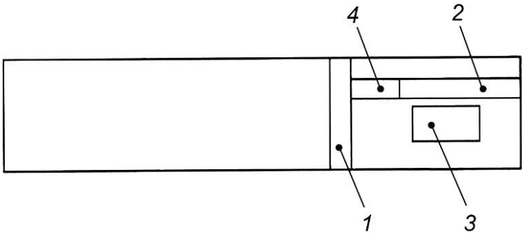
1 — кольцевая проба для контроля твердости [см. рисунок D.10 (приложение D), толщина не менее 6,4 мм (0,25 дюйма)]; 2 — проба для испытания на растяжение; 3 — проба для испытания на ударный изгиб [см. рисунок D.11 (приложение D)]; 4 — проба для контроля твердости [толщина не менее 6,4 мм (0,25 дюйма)], отбираемая от пробы для испытания на растяжение перед подготовкой образцов для испытаний
