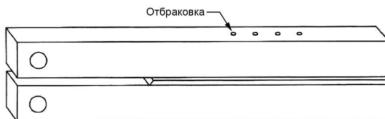
Рисунок D.30 — Расположение отпечатков при контроле твердости на образце DCB
