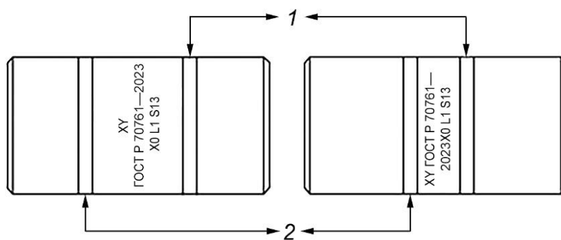
Рисунок D.29 — Пример расположения полос в цветовой маркировке муфты с уплотнительными кольцами
