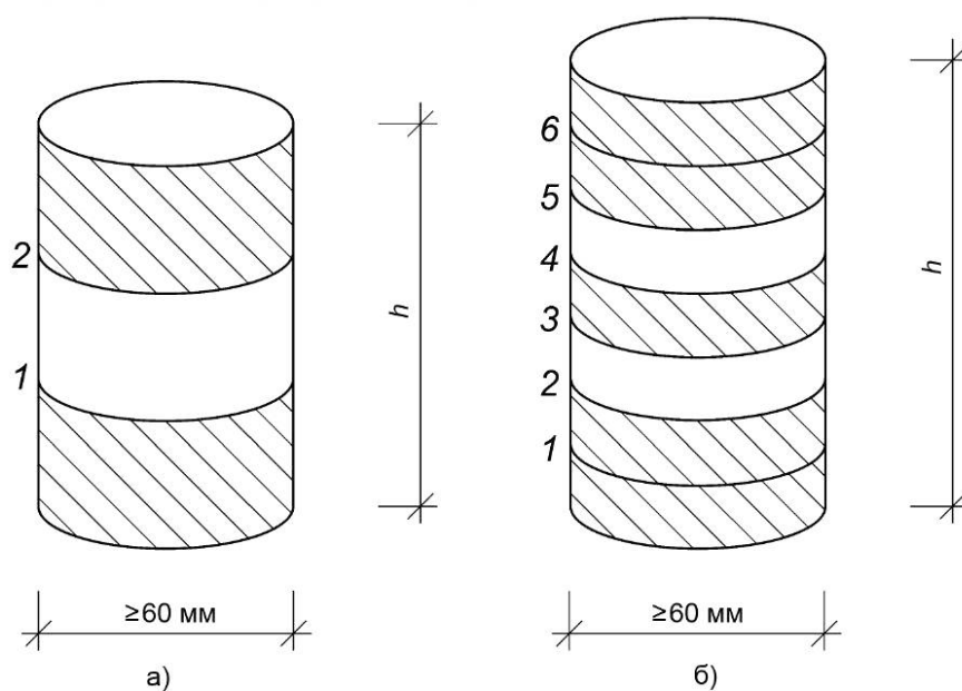
Рисунок 5 — Образцы для испытаний клеевых соединений слоев
