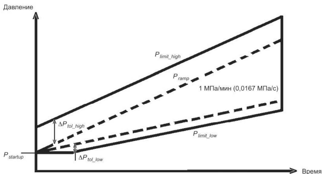
Рисунок 11 — Допуски по давлению для категории емкости СХКВ D
