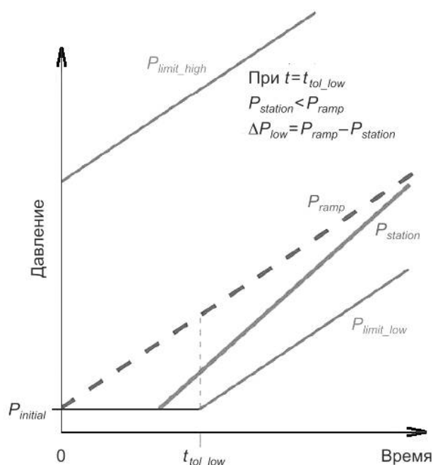
Рисунок И.12 — Иллюстрация отложенного начала заправки
