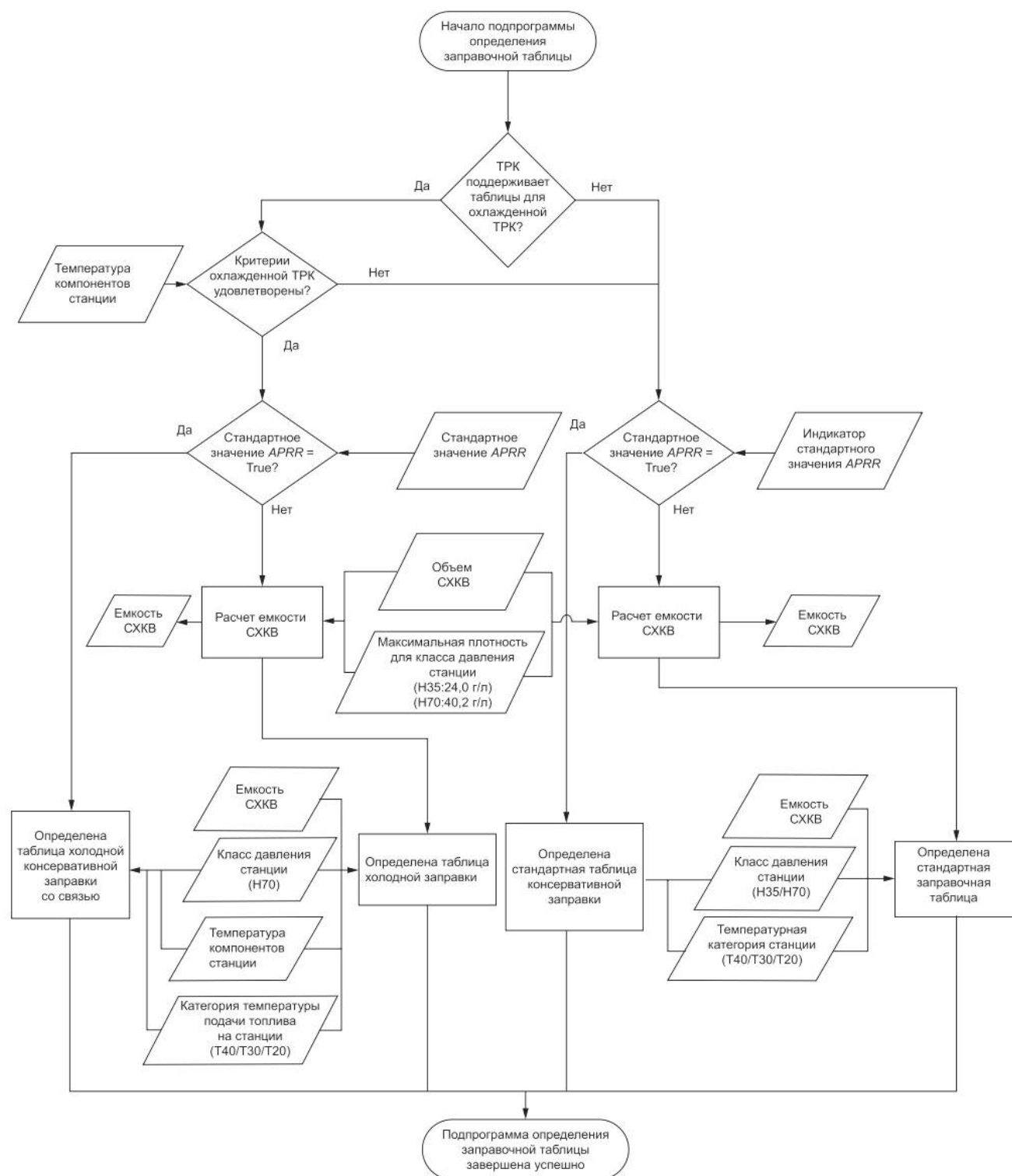
Рисунок Б.6 — Подпрограмма определения таблицы заправки
