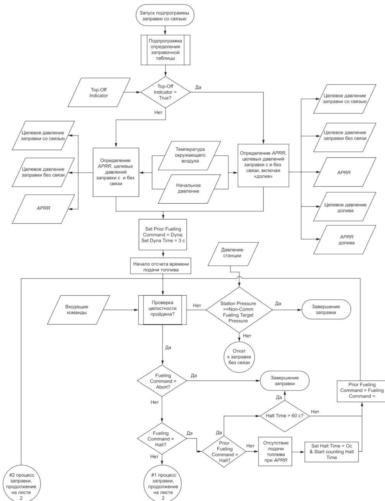
Рисунок Б.4 — Подпрограмма запуска заправки со связью
