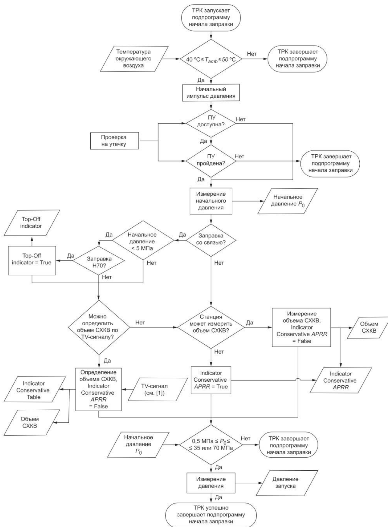
Рисунок Б.2 — Общая подпрограмма запуска ТРК
