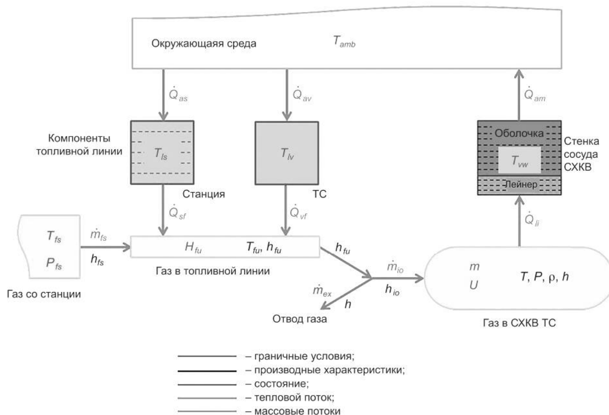
Рисунок А.1 — Имитационная модель
