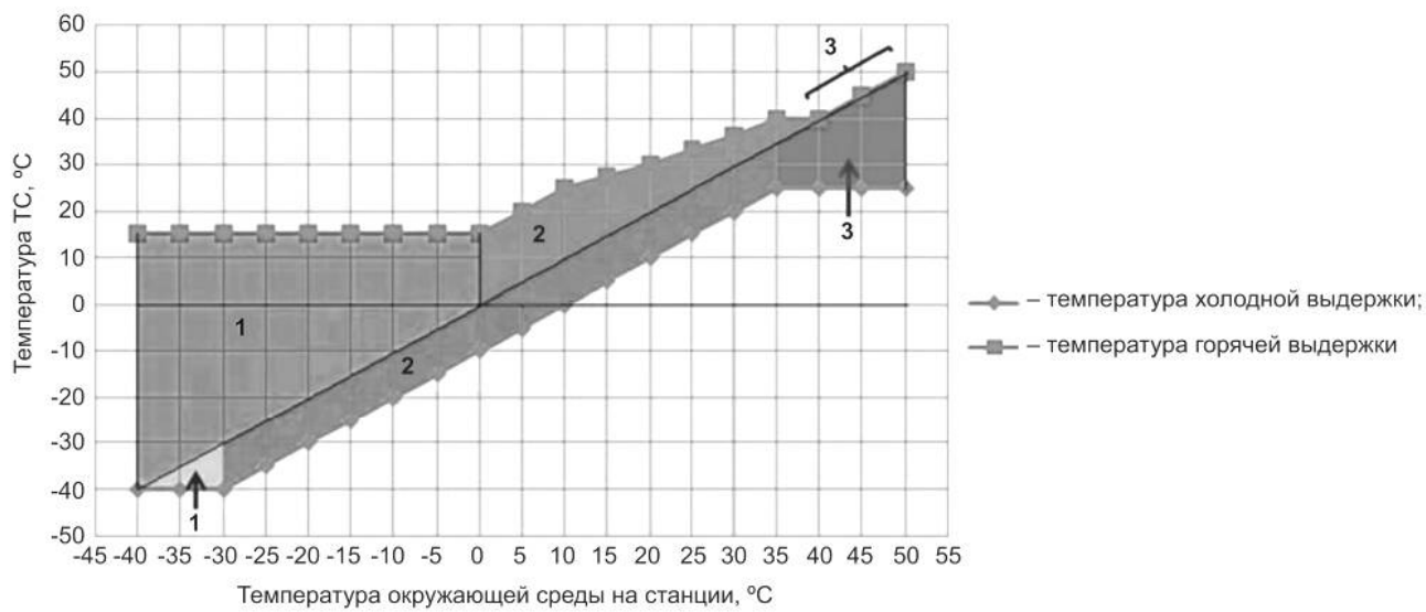
Рисунок А.5 — Положительные и отрицательные температурные отклонения СХКВ в зависимости от температуры окружающей среды
