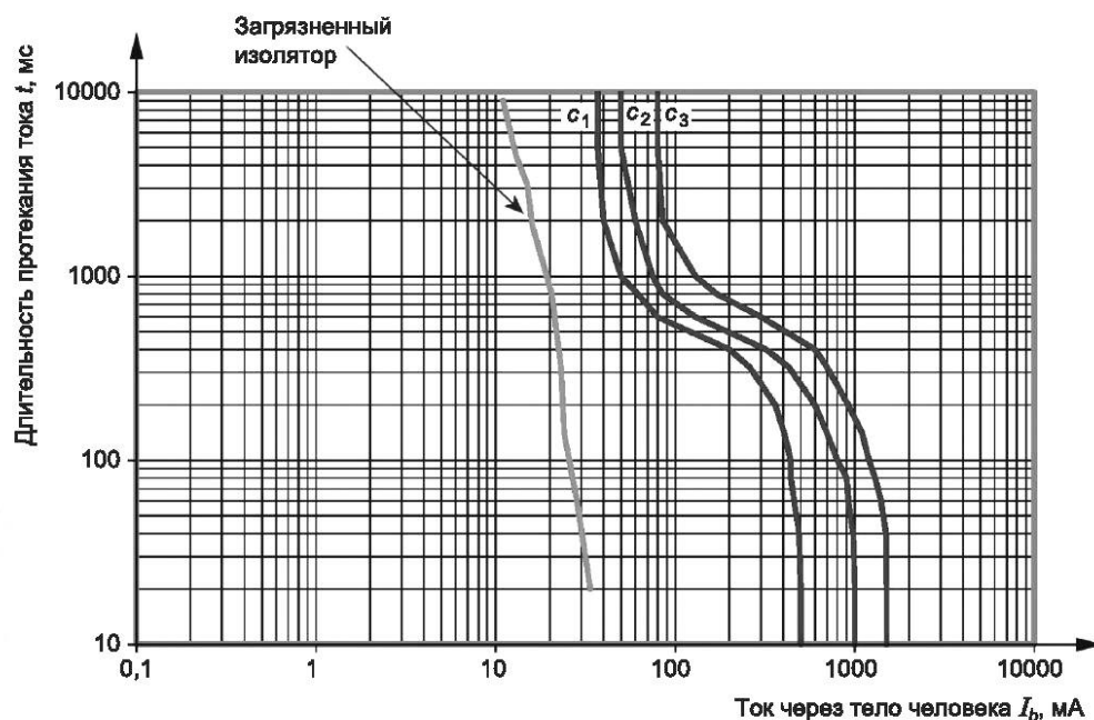
Рисунок 19 — Кривая BT, нанесенная на кривые зависимости тока от времени для переменного тока (см. рисунок A.19 ГОСТ Р 70646.1—2023)
