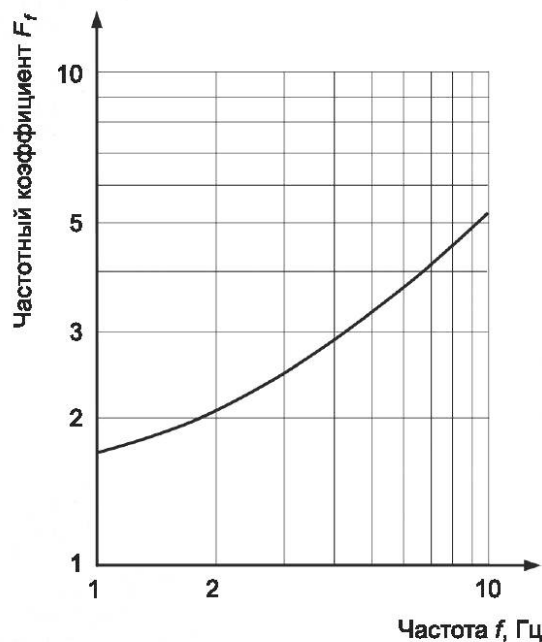
Рисунок 5 — Изменение порога отпускания для диапазона частот от 1000 до 10 000 Гц
