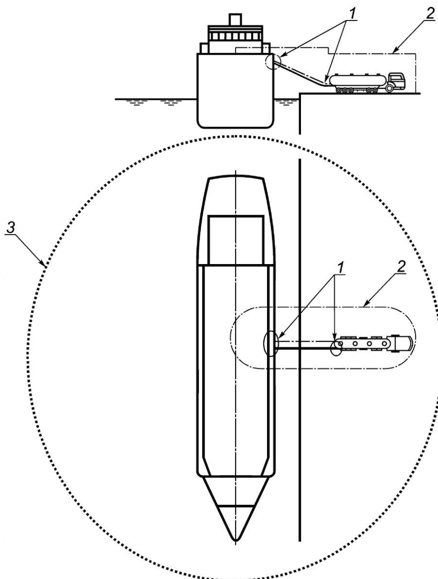
Рисунок А.1 — Опасная зона, зоны безопасности и зона мониторинга и охраны
