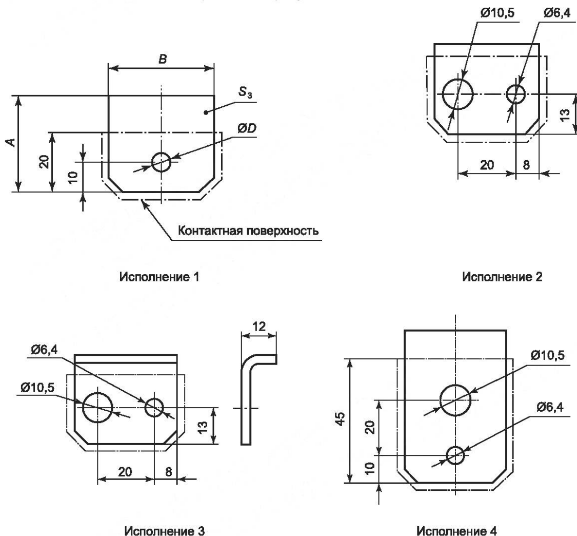
Рисунок 2 — Планки заземления
