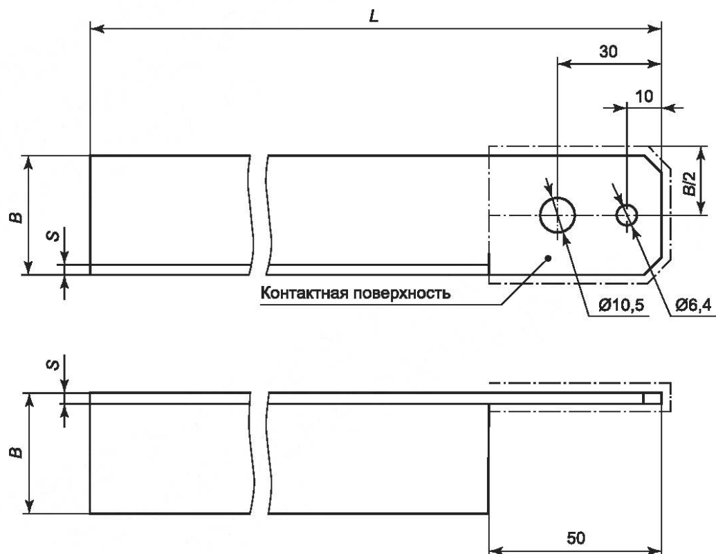
Рисунок 1 — Стойка заземления
