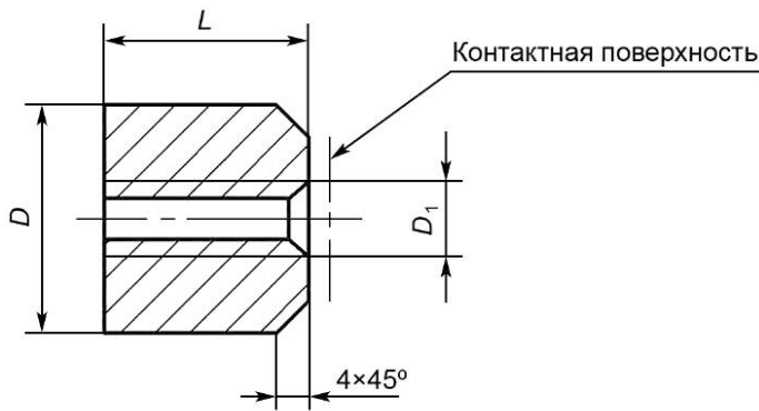
Рисунок 3 — Бонка заземления
