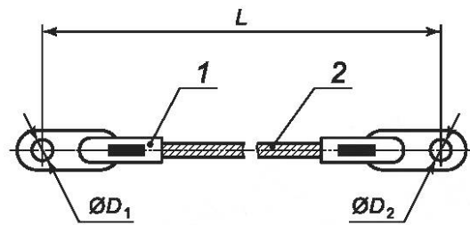
1 — наконечник; 2 — провод
