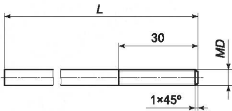
Рисунок 4 — Шпилька заземления
