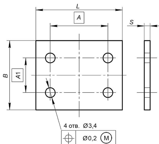
Рисунок 4 — Планка типа 2 для надписей общего применения
