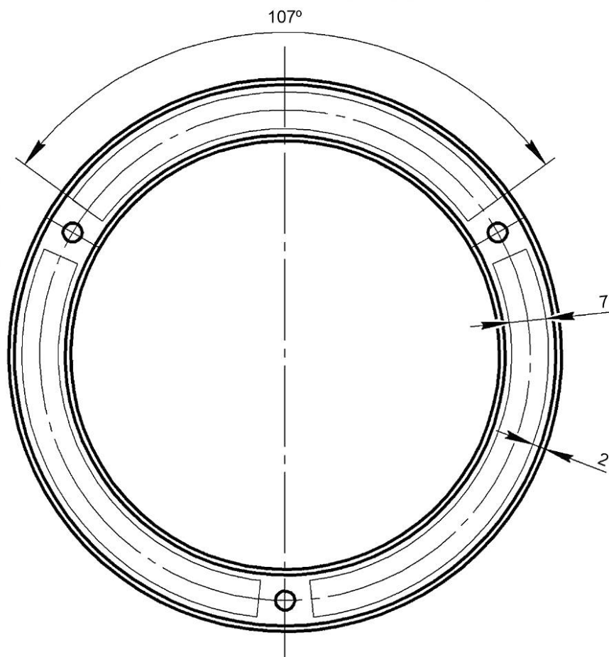
Рисунок И.1 — Расположение текстовых полей на планке типа 8
