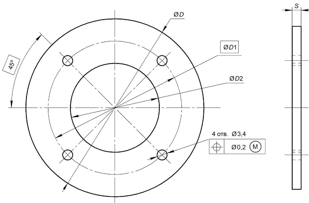
Рисунок 11 — Планка типа 6 для надписей к пакетным переключателям на три направления
