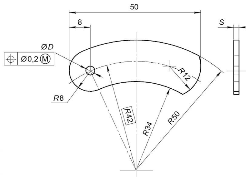
Рисунок 19 — Планка типа 10 для маркировки электроустановочной арматуры и светильников
