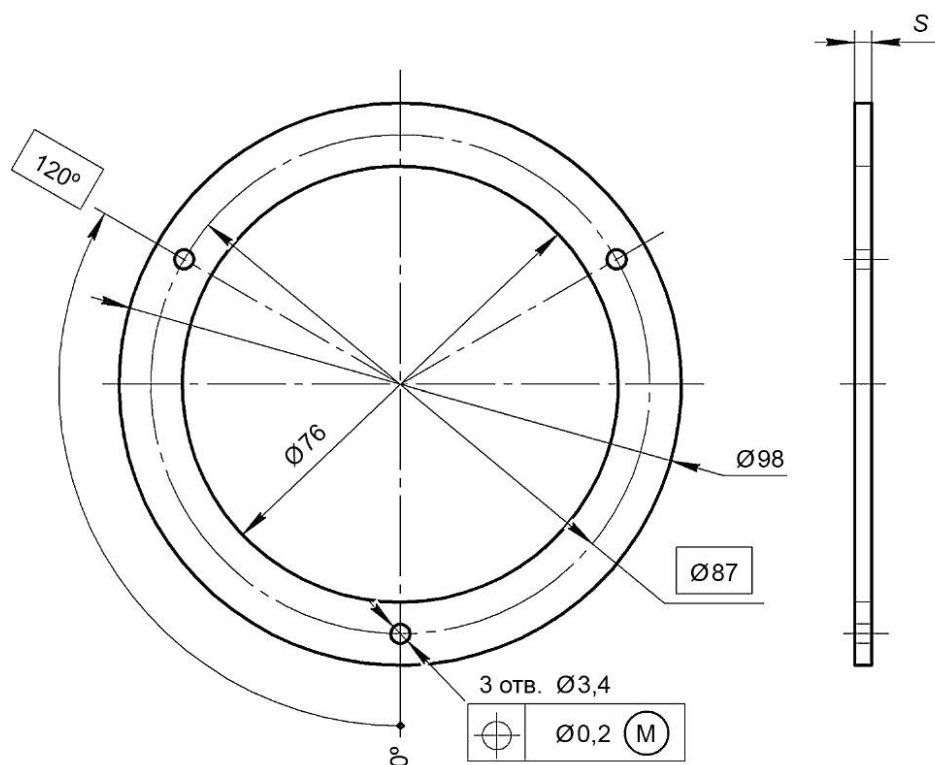
Рисунок 15 — Планка типа 8 для надписей к выключателям
