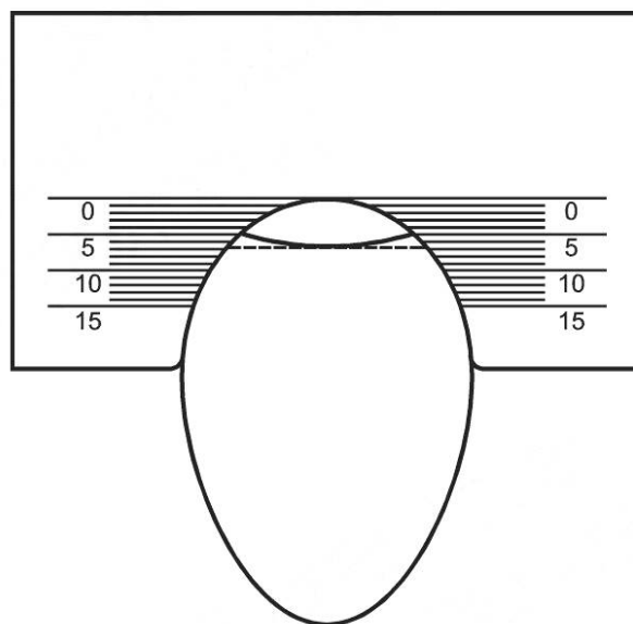
Рисунок 1 — Шаблон-измеритель для яиц, мм
