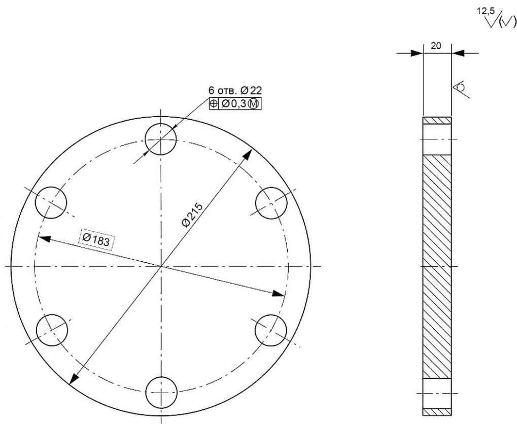
Рисунок 3 — Глухой фланец МФС НСВ
