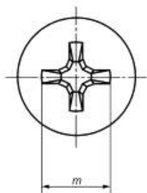
d) Крестообразный шлиц типа H
