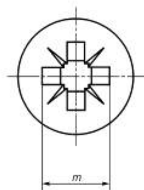
e) Крестообразный шлиц типа Z
