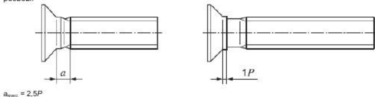
Рисунок 1 – Винт с подголовком для глубины вхождения серии 1 (глубокая)
