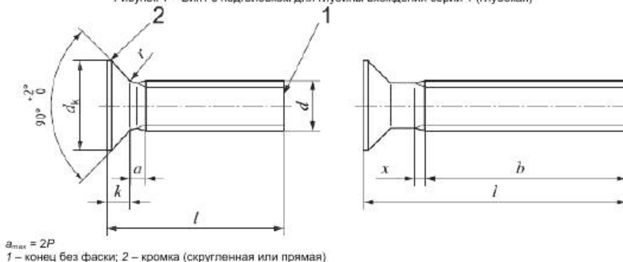
Рисунок 2 – Винт без подголовка для глубины вхождения серии 2 (мелкая)
