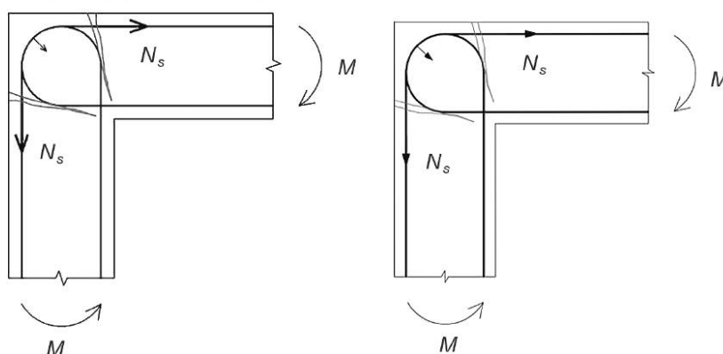
б) Тип Y-2 — угловой стык со сжатой внутренней гранью
