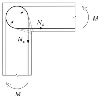
а) Тип Y-1 — угловой стык с растянутой внутренней гранью
