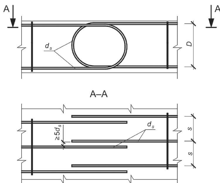
Рисунок 8.2 — Требование к расстоянию между петлями
