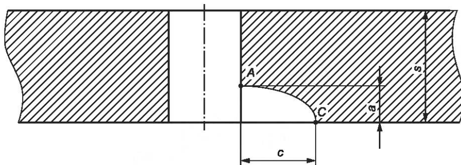
Рисунок 11.2 — Поверхностная четвертьэллиптическая трещина
