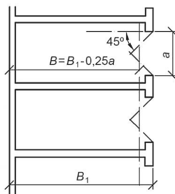
Рисунок 14 — К назначению расчетной ширины сооружения с анкерровкой контрфорсного типа
