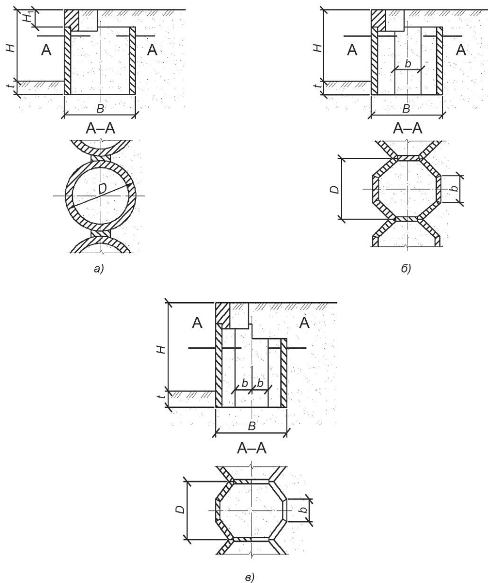
а) — из цилиндрических оболочек; б) и е) — полигональные из тонких железобетонных панелей
