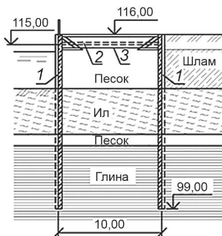
1 — стальной шпунт; 2 — анкерная тяга; 3 — распорка
