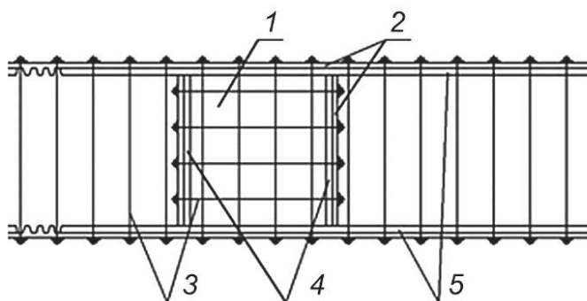
1 — блок усиления; 2 — распределительный пояс; 3 — анкерные тяги; 4 — поперечная шпунтовая стенка; 5 — продольная шпунтовая стенка
