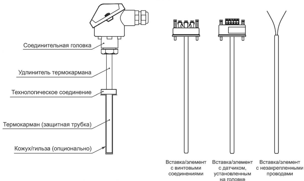
Рисунок 1 — Основные компоненты термоэлектрического/резистивного датчика температуры в сборе
