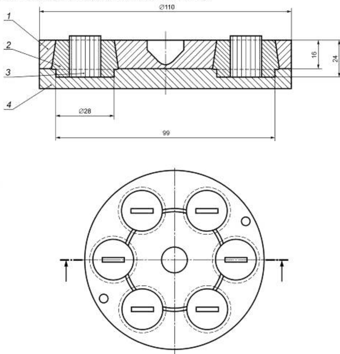
Рисунок 1 — Пример сборки для формования образцов
