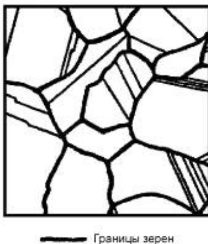
Рисунок 3 — Оценка числа зерен (зерна с двойниками)
