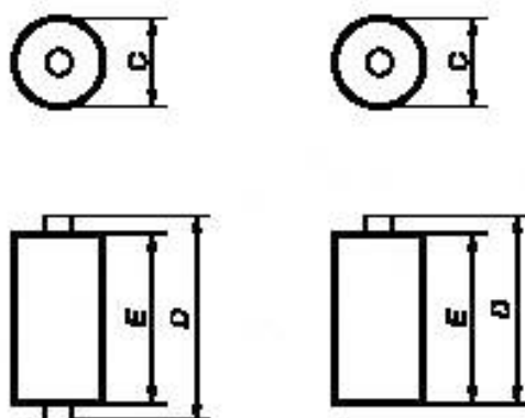
Рисунок 1 — Примеры измерений максимальных размеров цилиндрического аккумулятора
