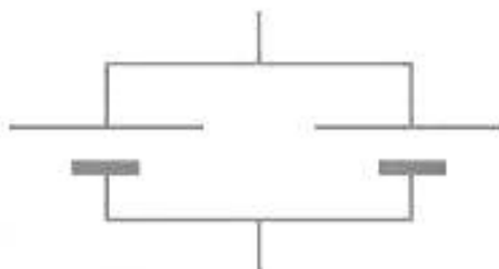
Рисунок А.2 — Архитектура построения батареи 2P
