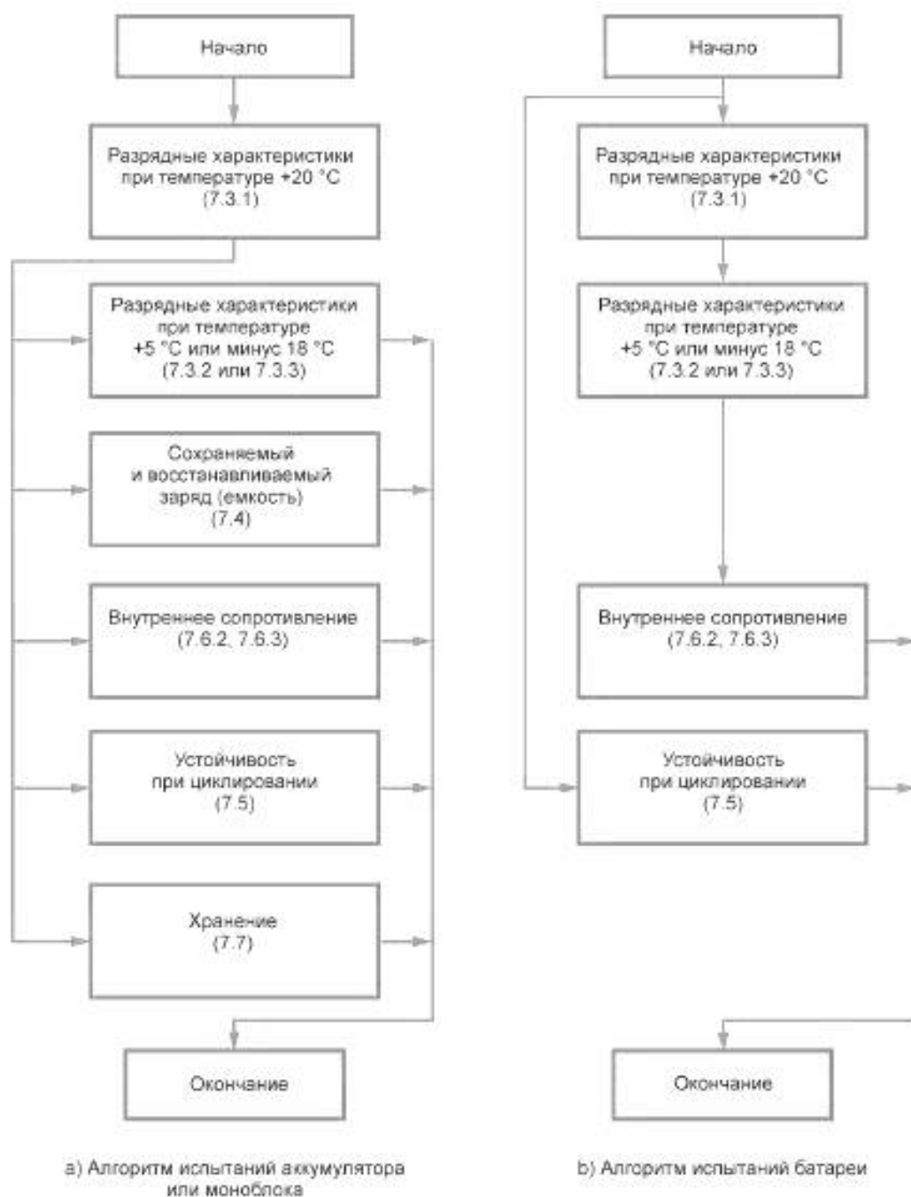
Рисунок 3 — Алгоритм испытаний
