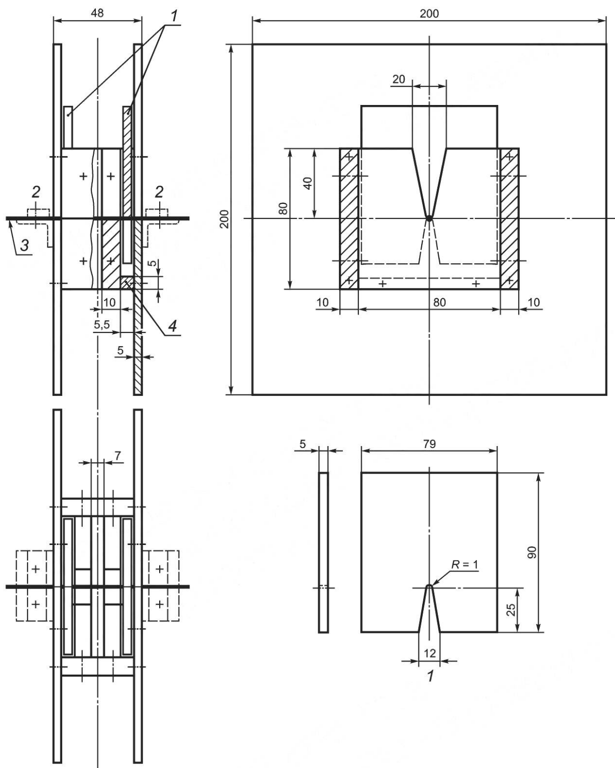
Рисунок 10 — Испытательная установка для проверки минимальных значений R^2t и I_p , которые должно выдерживать устройство RDC-DD [9.11.2.1 а)]
