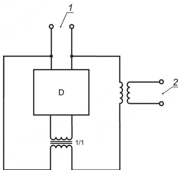
Рисунок 23 — Пример испытательной цепи для проверки старения электронных компонентов (9.20)
