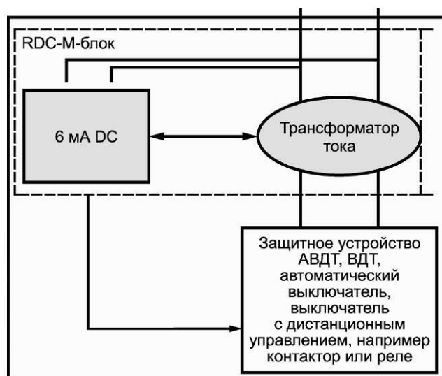
Рисунок L.3 — Устройство RDC-MD согласно классификации 4.1.1.3 (с электрическим соединением)
