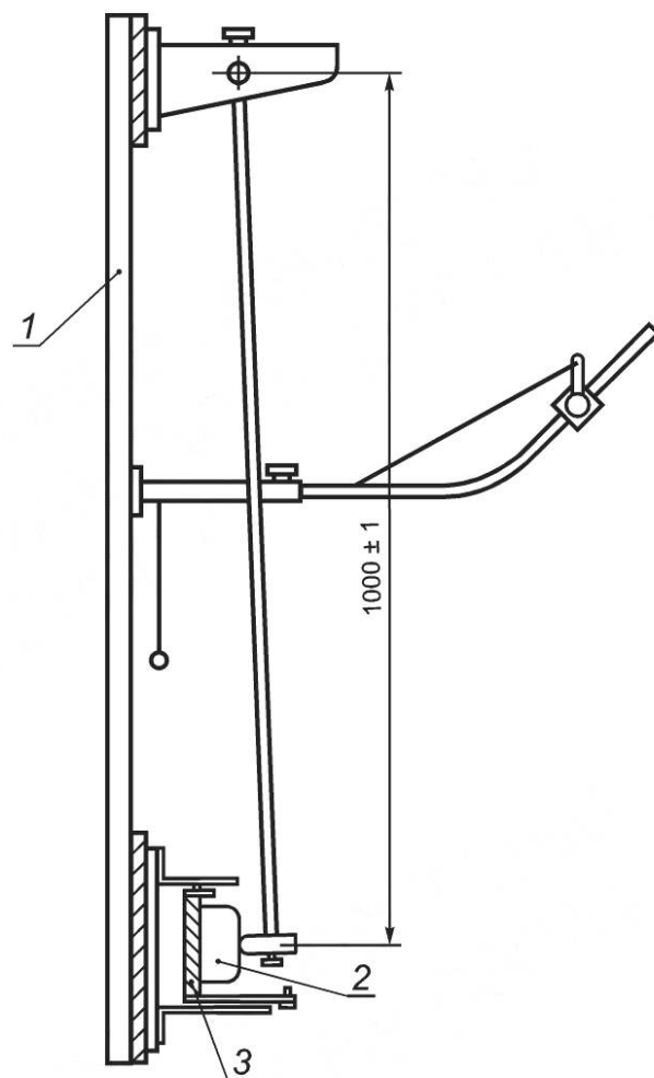
Рисунок 12 — Испытательная установка для испытания прочности на удар (9.12.2.1)
