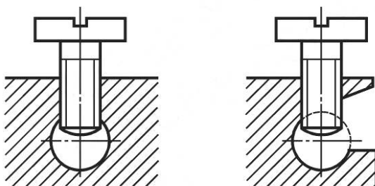
b) Зажимы без прижимных пластин
