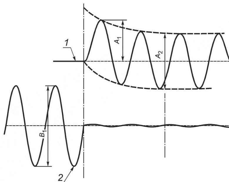
Рисунок 26 — Пример записи калибровки для испытания на короткое замыкание [9.11.2.1 j) 1)]
