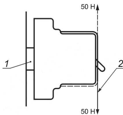
1 — рейка; 2 — проволока
