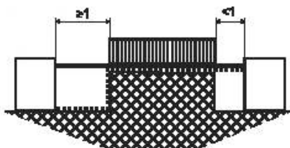
Рисунок А.1b — Зазор для ребра и бесклеевого стыка с пазом
