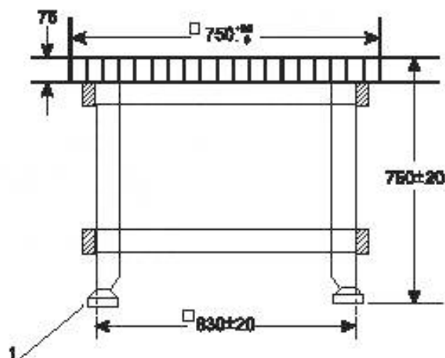
Рисунок I.1 — Испытательная стойка
