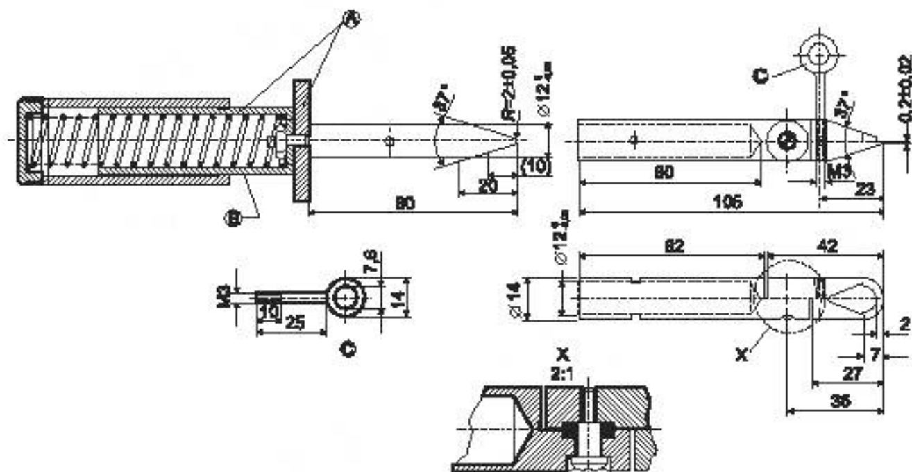
Рисунок 1 — Испытательный ноготь
