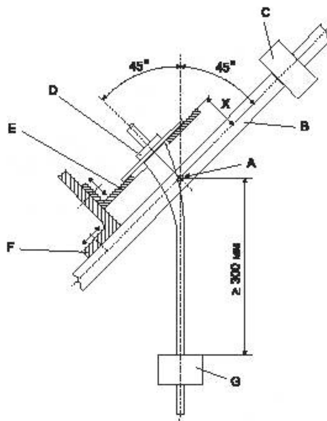
A — ось качения; B — качающаяся рама; C — противовес; D — образец; E — регулируемая опорная плита; F — регулируемый кронштейн; G — груз
