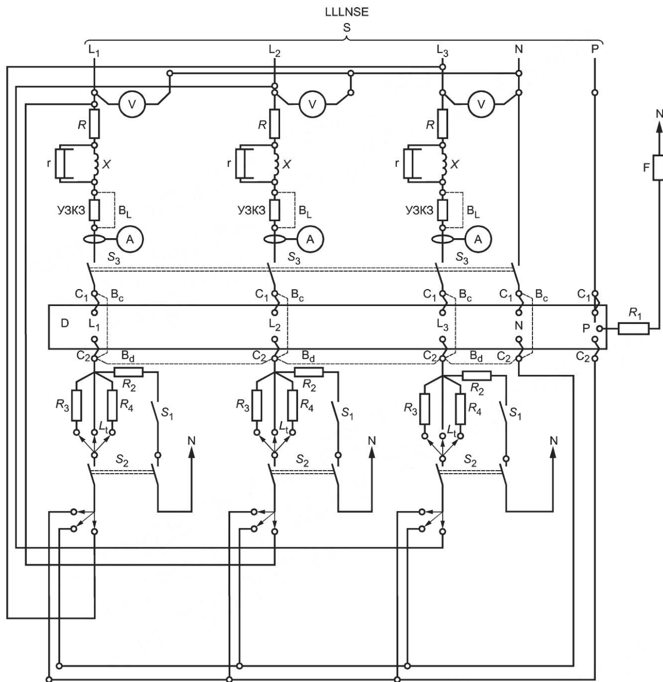
с) Тип LLLNSE/LLNE
