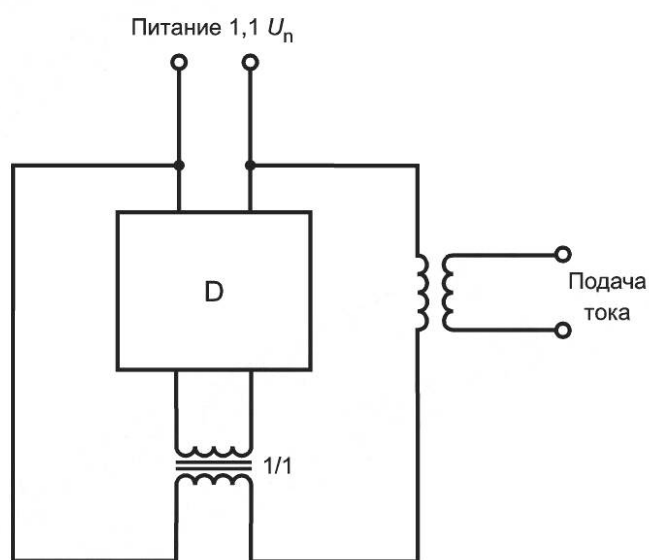
Рисунок 21 — Цикл испытаний надежности (9.17.1.4)
