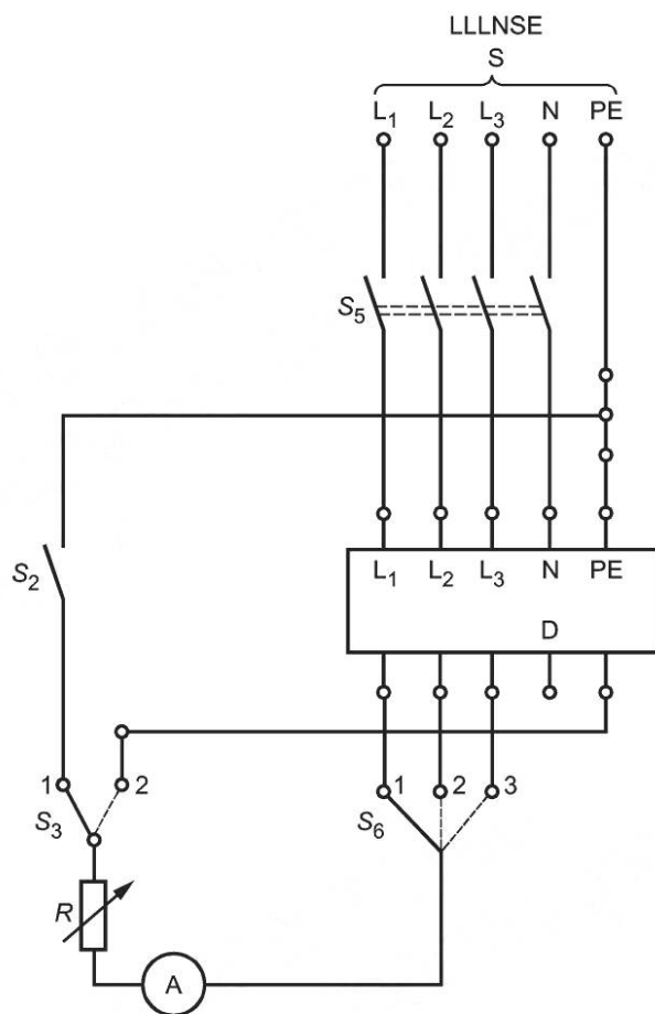
с) Тип LLLNSE/LLLNE
