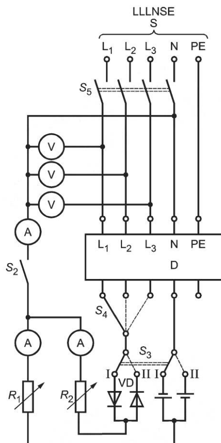
с) Типы LLLNSE/LLLNE
