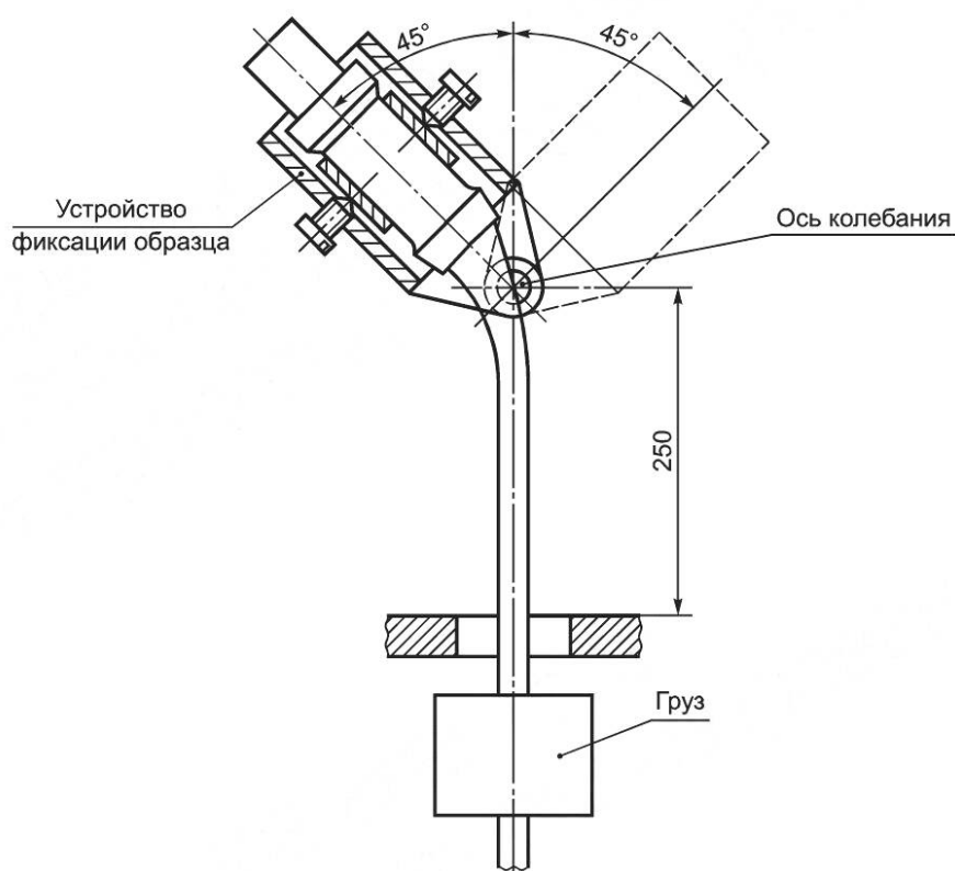
Рисунок 17 — Устройство для испытания натяжения провода
