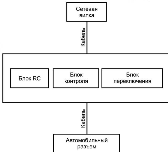
Рисунок Е.1 — Пример IC-CPD с разными частями и функциями
