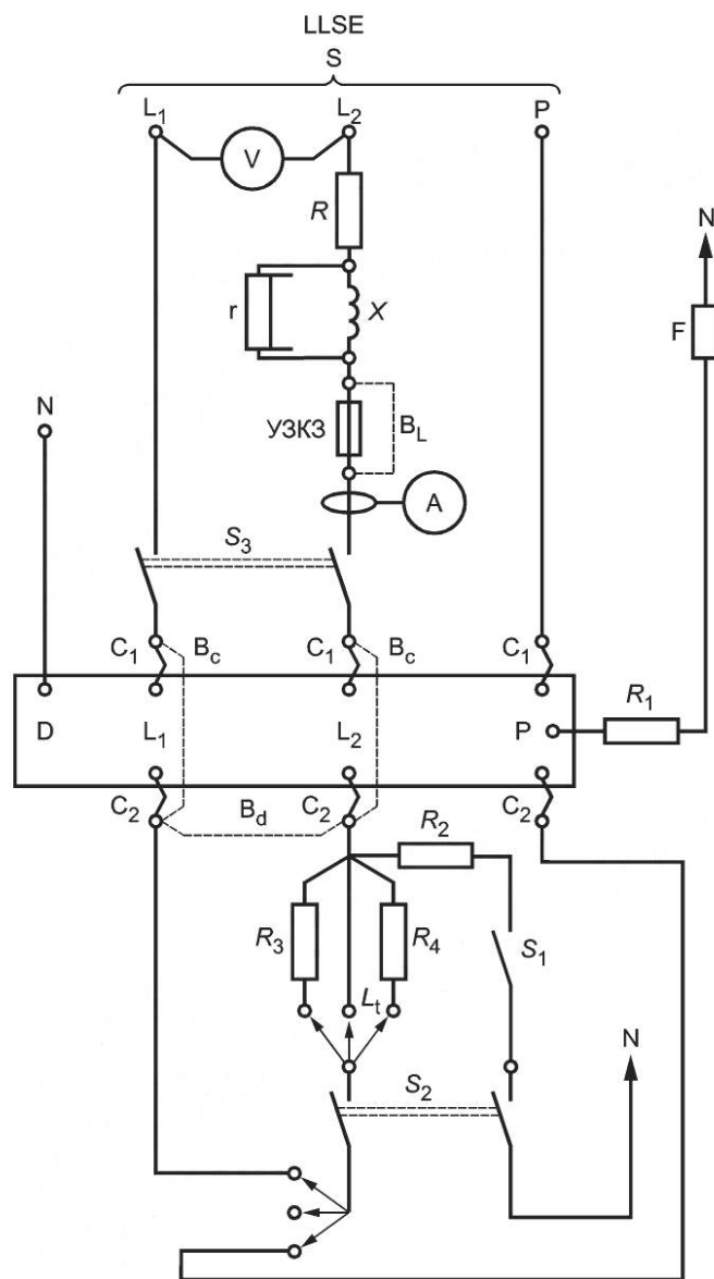
b) Тип LLSE/LLE
