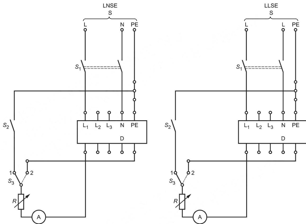
с) Тип LLLNE/LLLNE в сети LNSE
