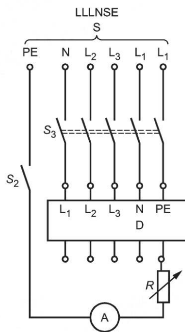
h) Тип LLLNSE
