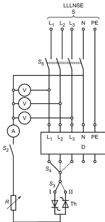
с) Типы LLLNSE/LLNE
