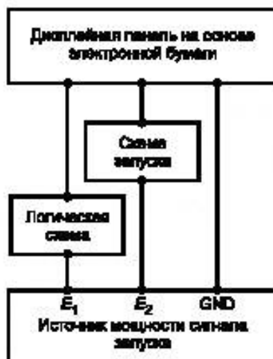
Рисунок 1 — Блок-схема для разьяснения напряжения питания
