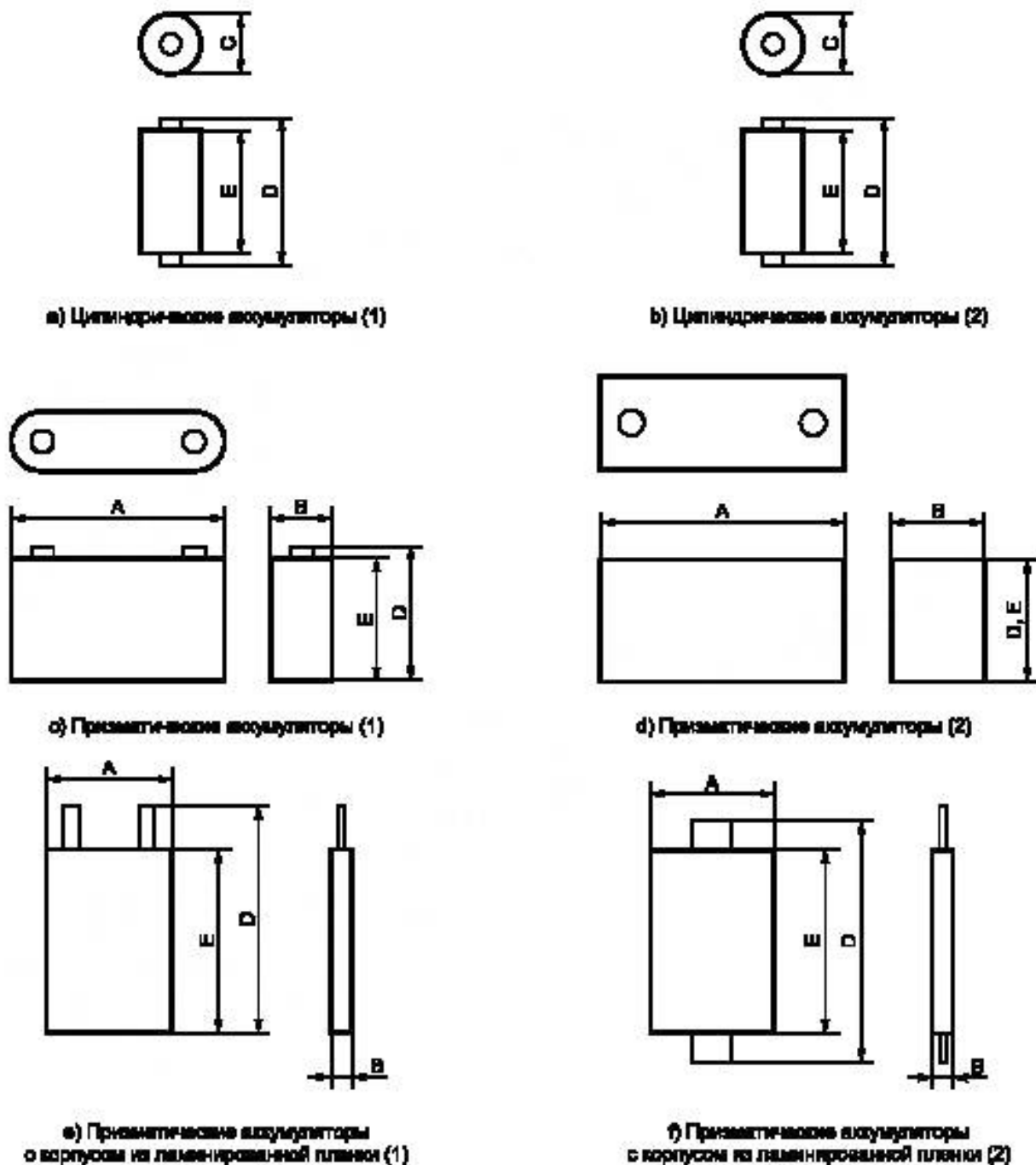
Рисунок 2 — Примеры измерений габаритных размеров аккумуляторов
