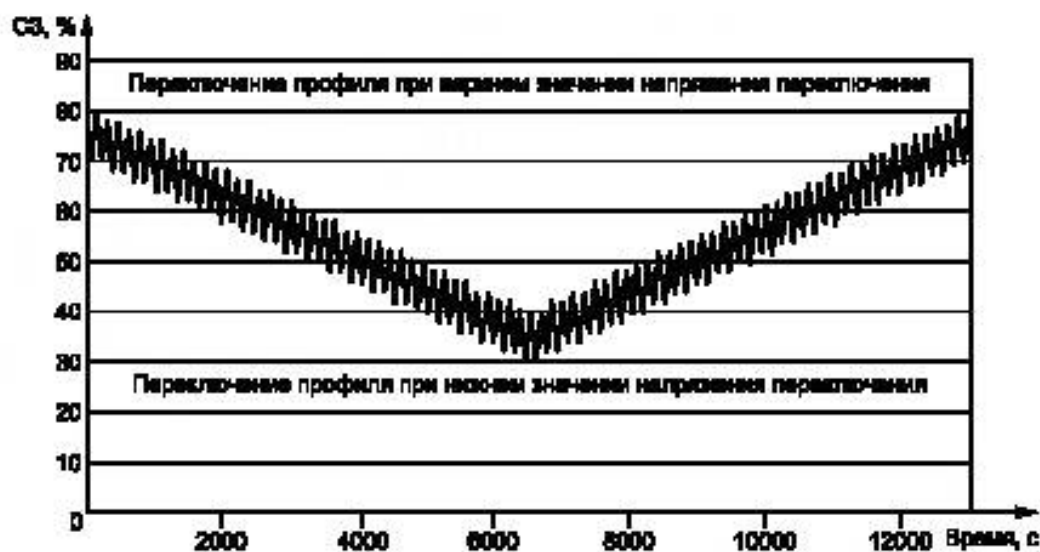
Рисунок 7 — Типичное колебание C3 в режиме двух последовательных профилей при циклировании аккумуляторов для ЭМГ
