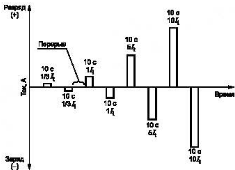
а) Порядок проведения испытания по определению ВАХ для применения ЭМГ
