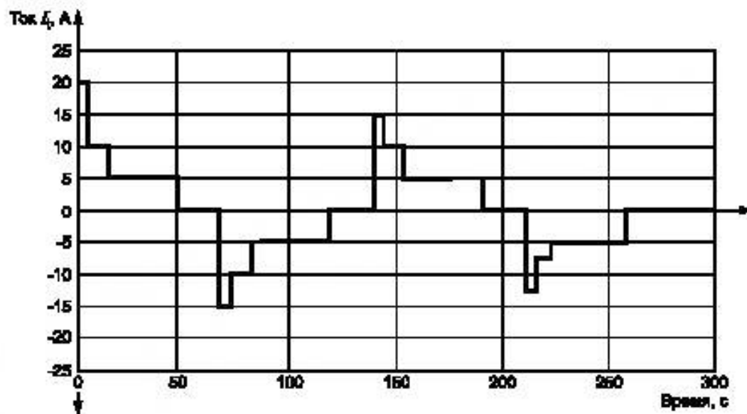
Рисунок 5 — ППР при циклировании аккумуляторов для ЭМГ
