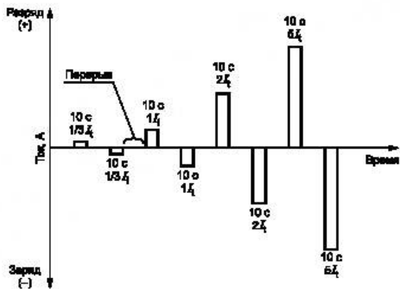
б) Порядок проведения испытания по определению ВАХ для применения ЭМА
