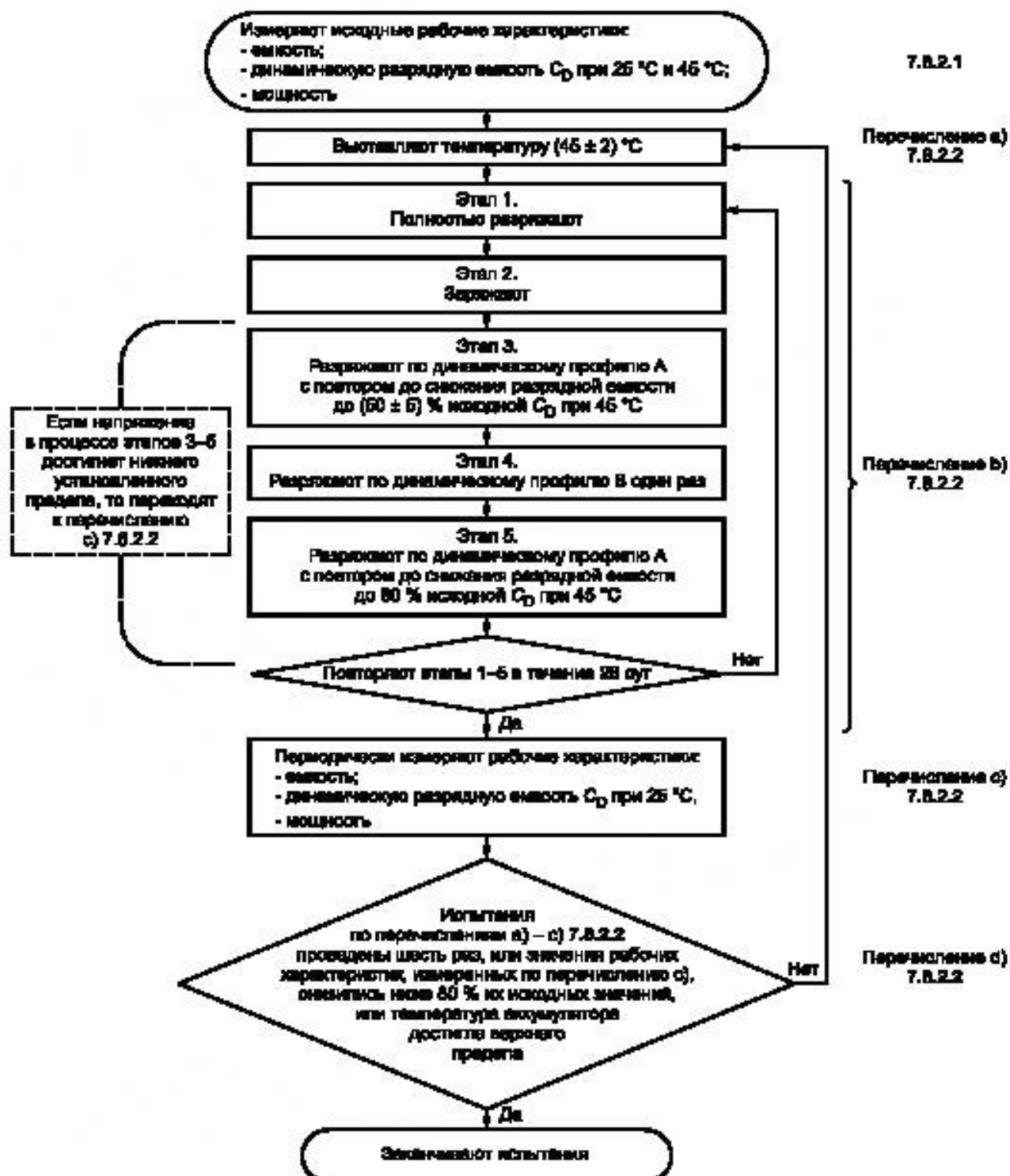
Рисунок В.1 — Последовательность испытаний при циклировании аккумуляторов для ЭМА
