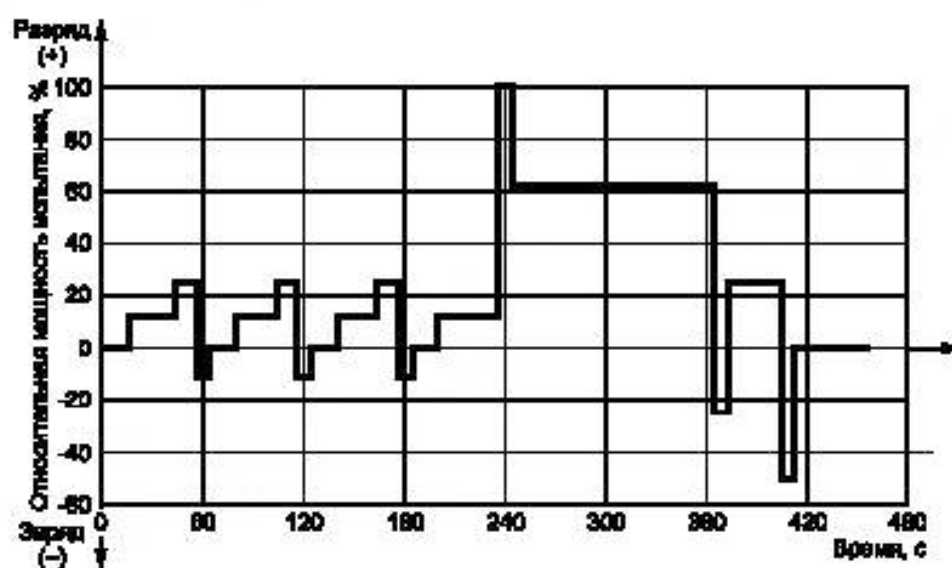
Рисунок 4 — Динамический разрядный профиль В циклирования аккумуляторов для ЭМА
