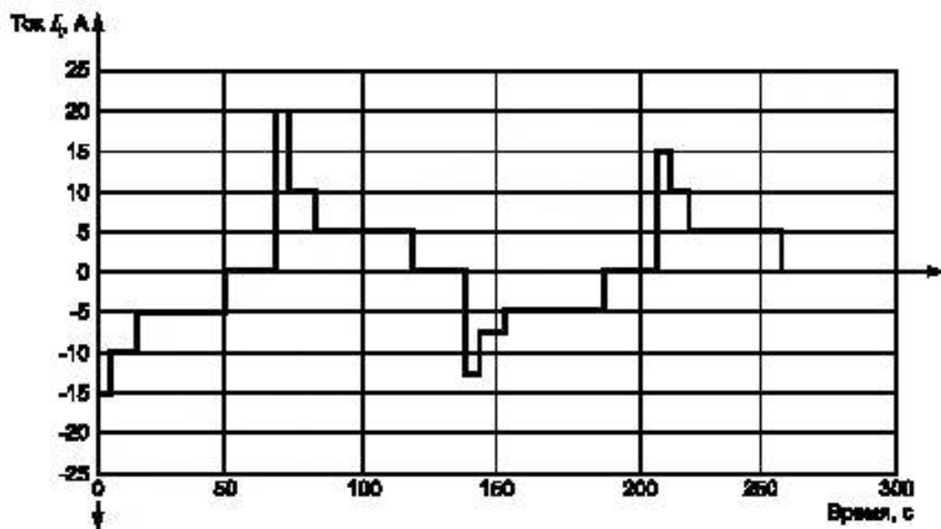
Рисунок 6 — ППЗ при циклировании аккумуляторов для ЭМГ
