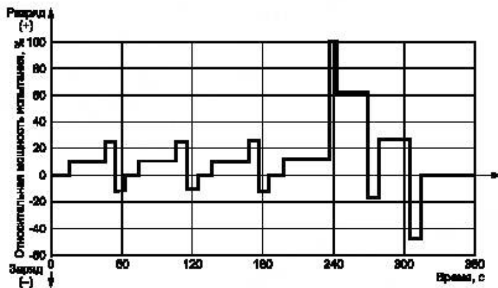
Рисунок 3 — Динамический разрядный профиль А циклирования аккумуляторов для ЭМА
