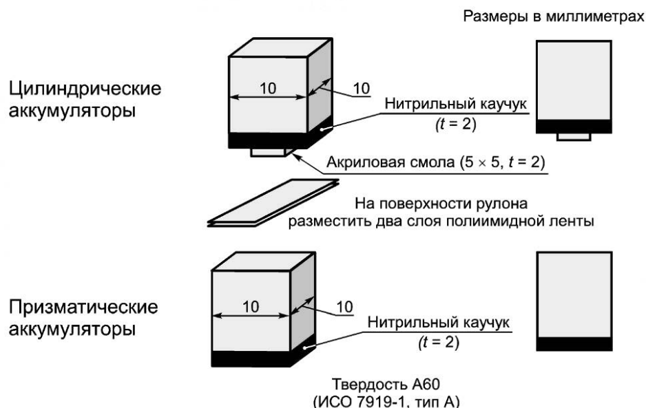
Рисунок 5 — Приспособление для нажатия 1)
