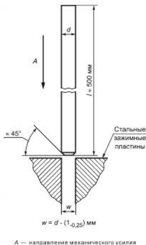
Рисунок 2 — Пример испытания адгезии
