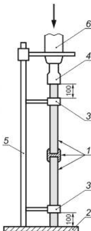
1 — образец; 2 — металлическая плита; 3 — подшпик; 4 — приводная головка; 5 — стойка испытательной установки; 6 — вибрационный молот
