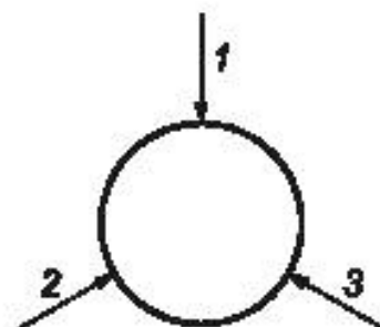
Рисунок 1 — Пример измерения толщины покрытия по окружности стержня
