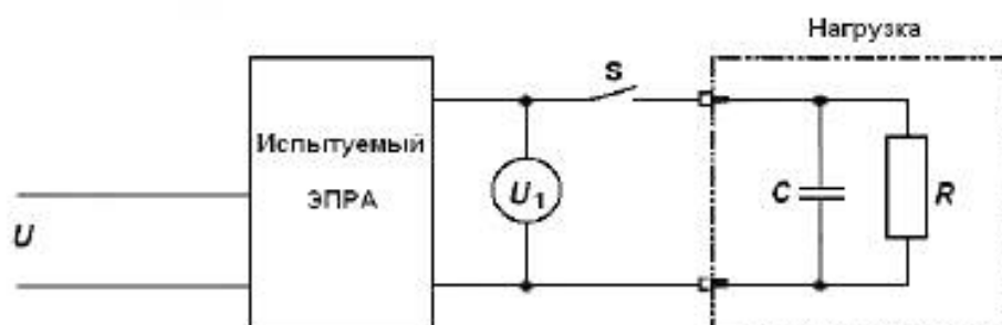
Рисунок A.1b — Испытательная схема измерения тока при соединении ЭПРА с нагрузкой после достижения установившегося режима работы
