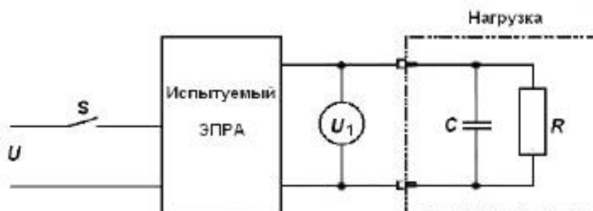
Рисунок A.1a — Испытательная схема измерения тока при включении ЭПРА в сеть
