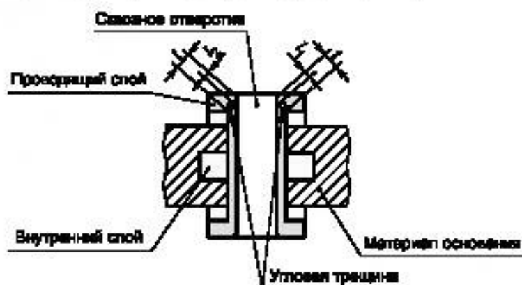
Рисунок 39 — Угловая трещина
