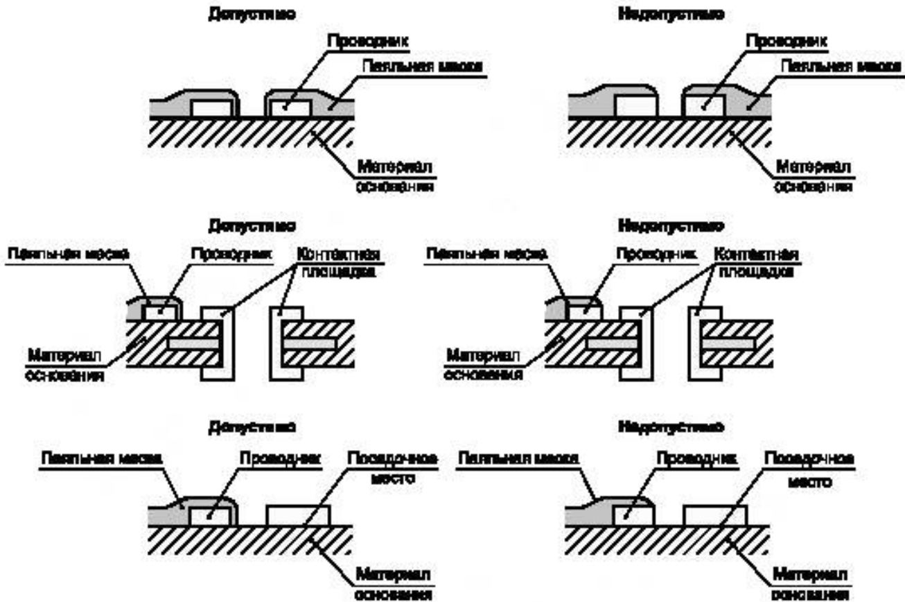
Рисунок 22 — Изображение проводника
