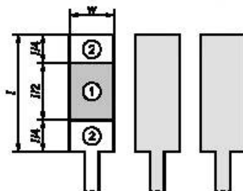
Рисунок 33 — Проверяемые области дефектов печатного контакта
