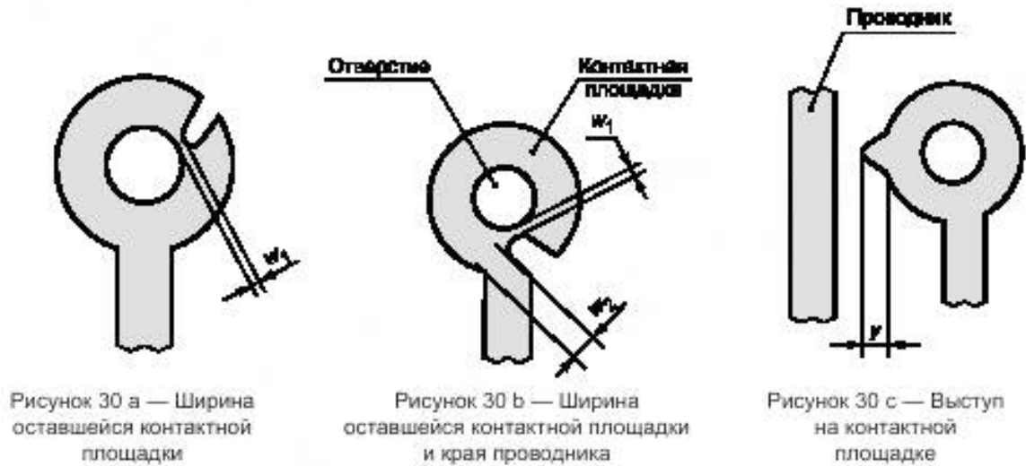
Рисунок 30 — Контактная площадка
