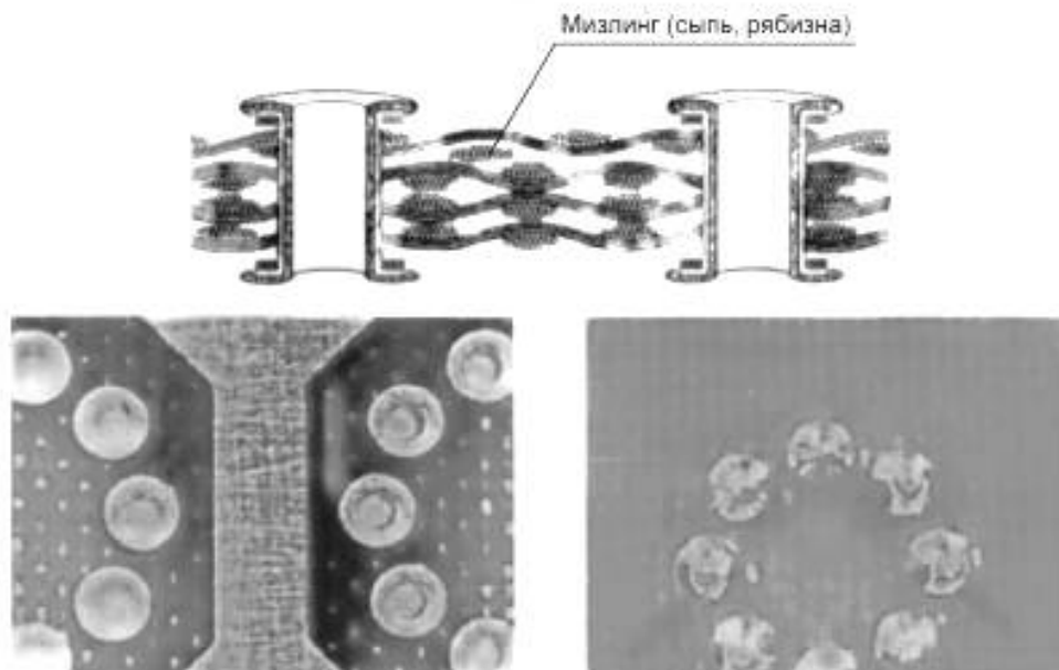
Рисунок 26 — Пример мизлинга
