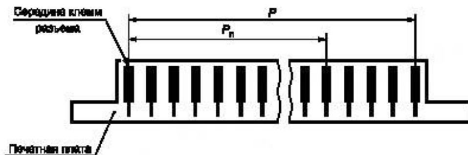
Рисунок 13 — Расстояние между серединами клемм
