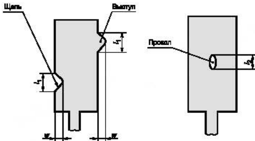
Рисунок 34 а — Щель и выступ
