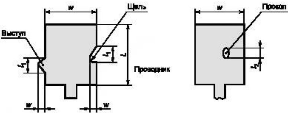
Рисунок 31 — Дефекты на контактной площадке посадочного места
