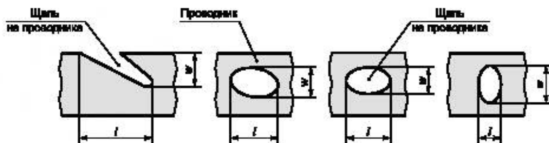
Рисунок 28 — Щели проводников
