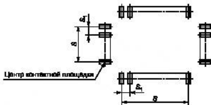
Рисунок 16 — Посадочное место
