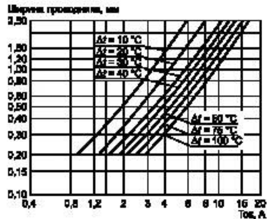
Рисунок 36 в — толщина проводника составляет 70 мкм
