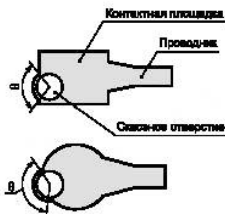
Рисунок 21 с — Допустимая область разрыва пояса
