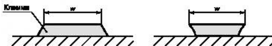
Рисунок 14 — Ширина клемм
