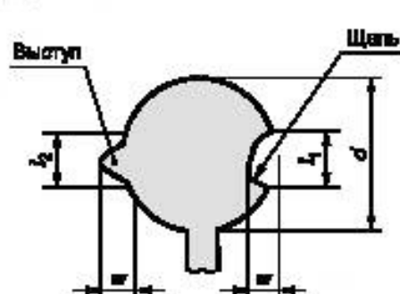
Рисунок 32 а — Щель и выступ
