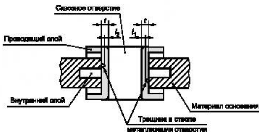
Рисунок 40 — Трещина ствола
