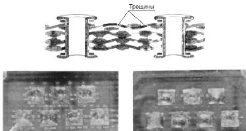
Рисунок 27 — Примеры трещин
