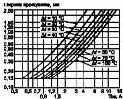
Рисунок 36 б — толщина проводника составляет 35 мкм
