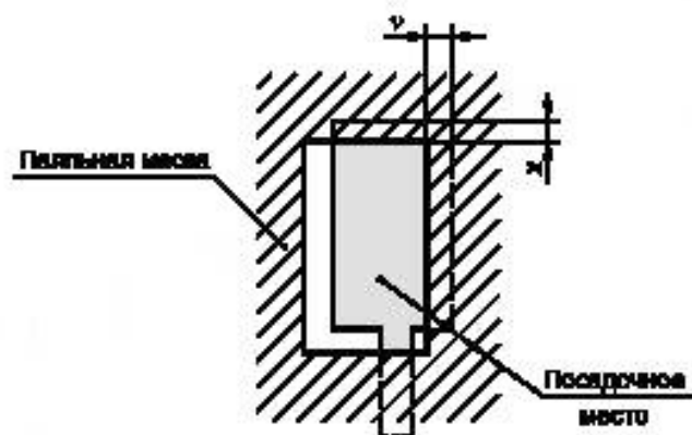
Рисунок 24 а — Смещение паяльной маски
