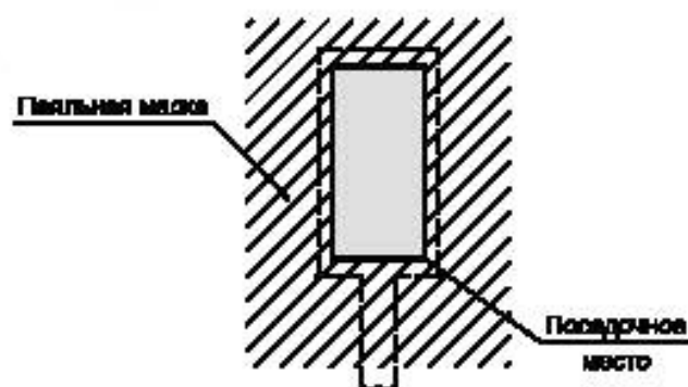
Рисунок 24 б — Смещение и полное покрытие паяльной маской
