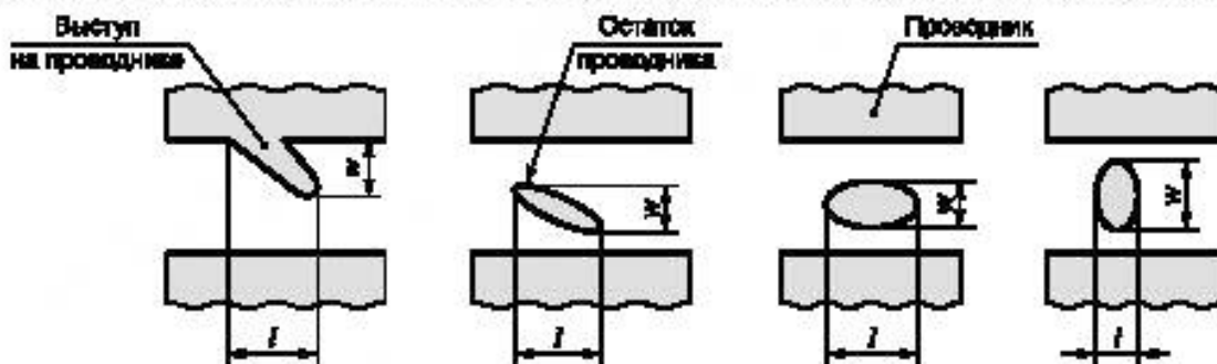
Рисунок 29 — Остаток проводника
