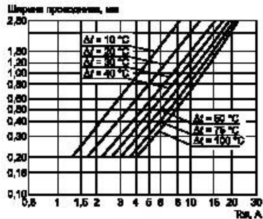
Рисунок 36 д — толщина проводника составляет 105 мкм
