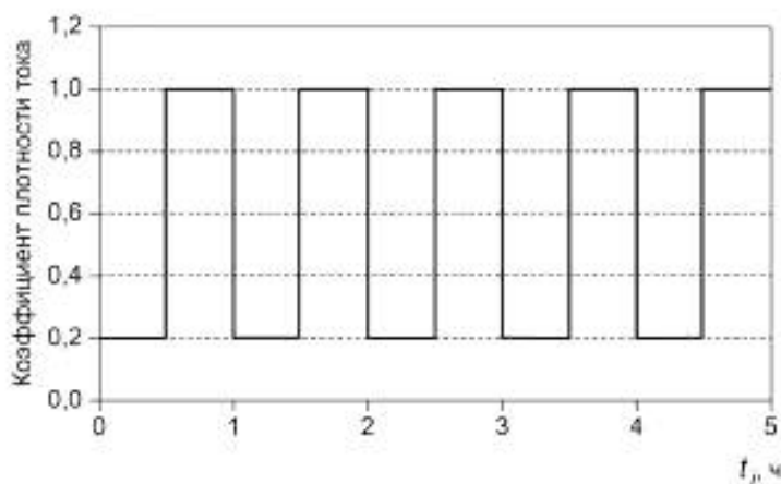
Рисунок I.2 — Второй профиль циклического изменения нагрузки
