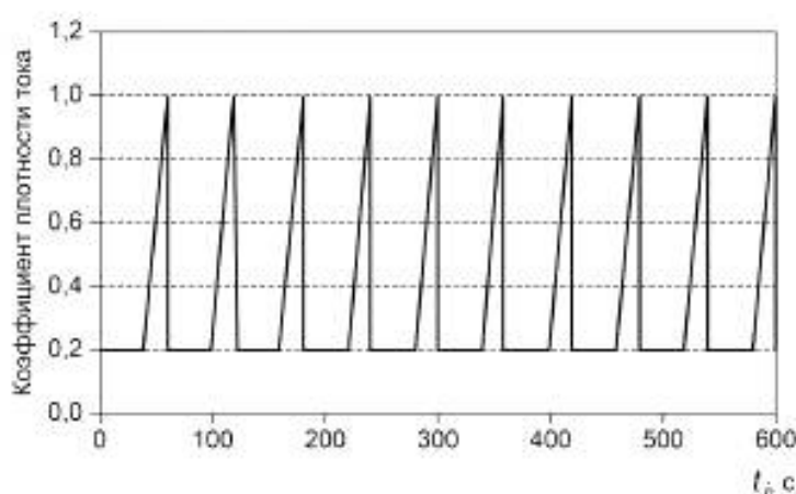
Рисунок I.1 — Первый профиль циклического изменения нагрузки
