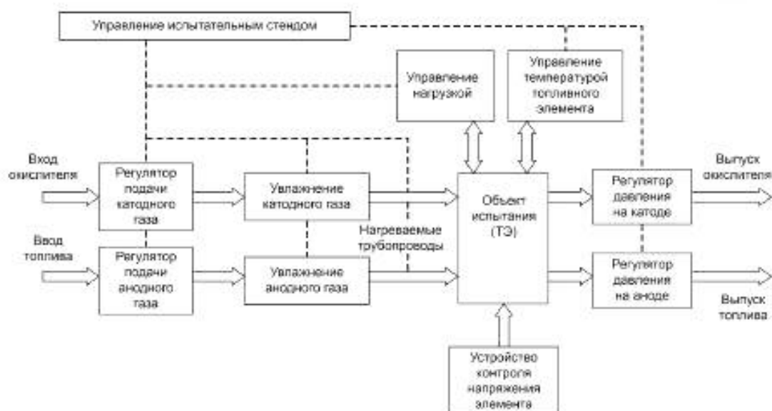
Рисунок 1 — Принципиальная схема стенда для испытания единичного элемента
