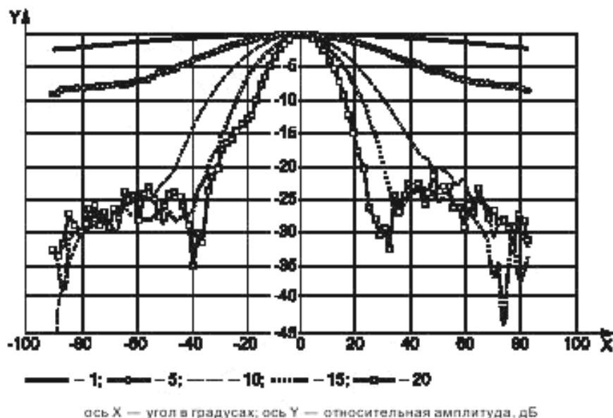
Рисунок А.2 — Характеристики направленности 0,2 мм — зондового гидрофона
