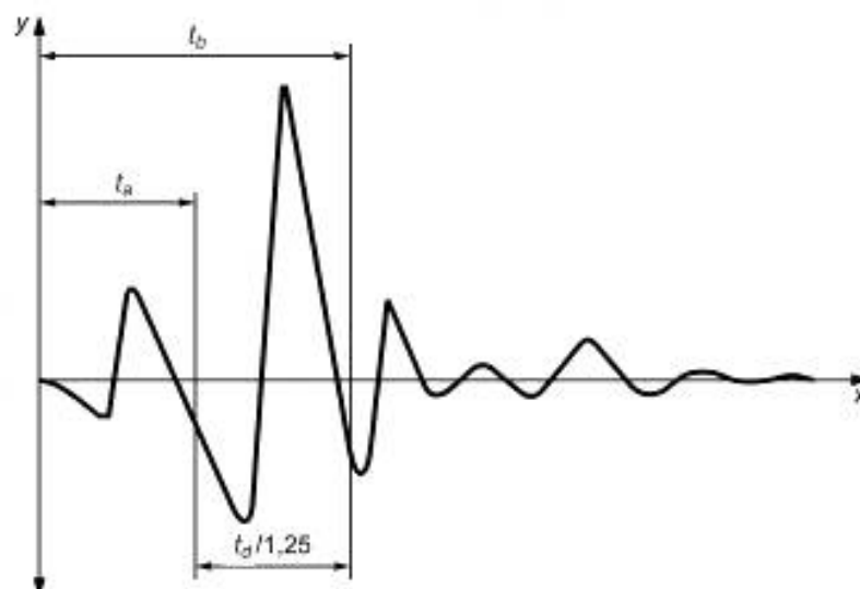
Рисунок 2 — Определение длительности импульса t_d
