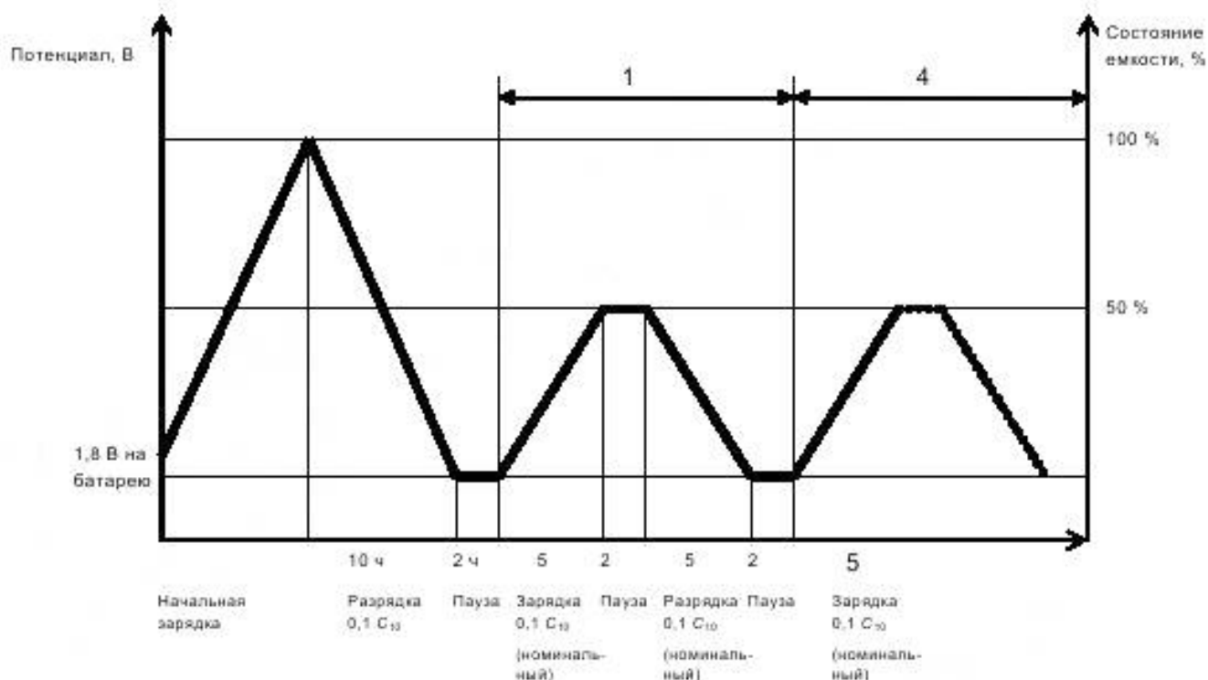
Рисунок 2 — Циклические условия эффективности метода испытаний
