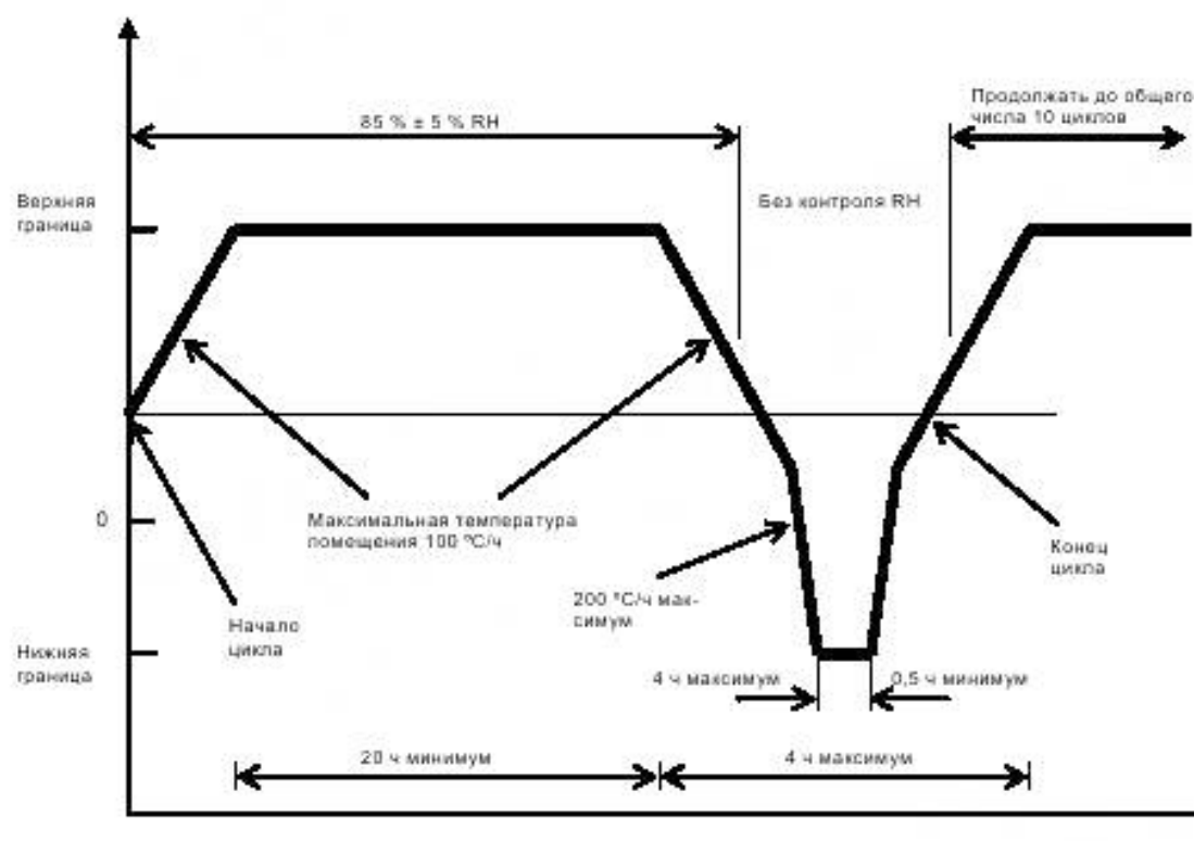
Рисунок 5 — Испытание на стойкость к влажности и низким температурам
