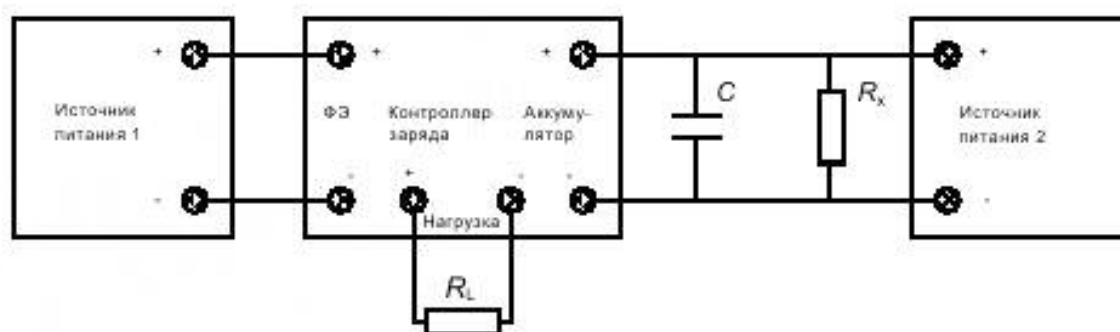
Рисунок 3 — Схема проверки без подключения измерительных приборов
