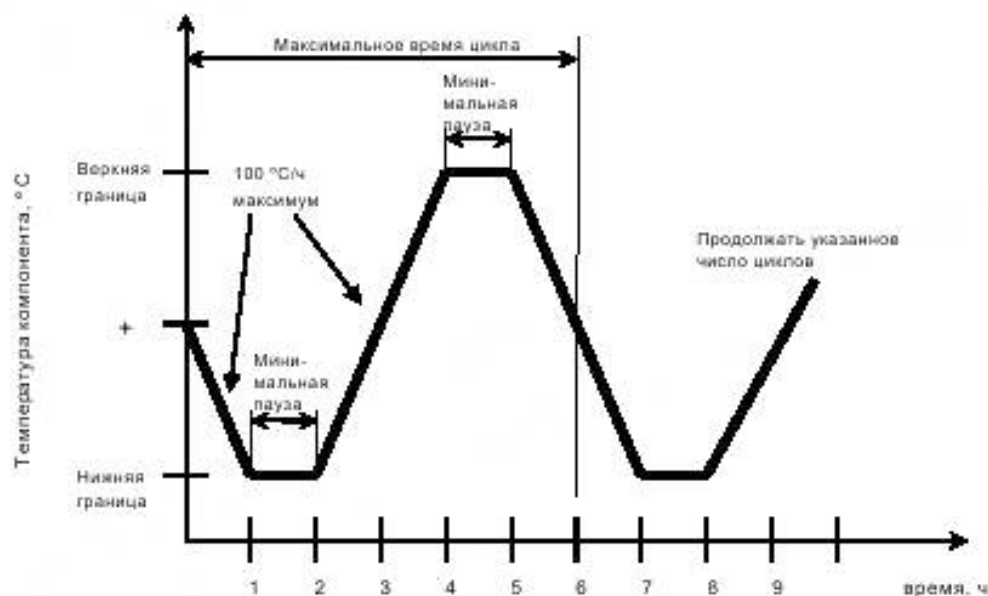
Рисунок 4 — Термоциклирование
