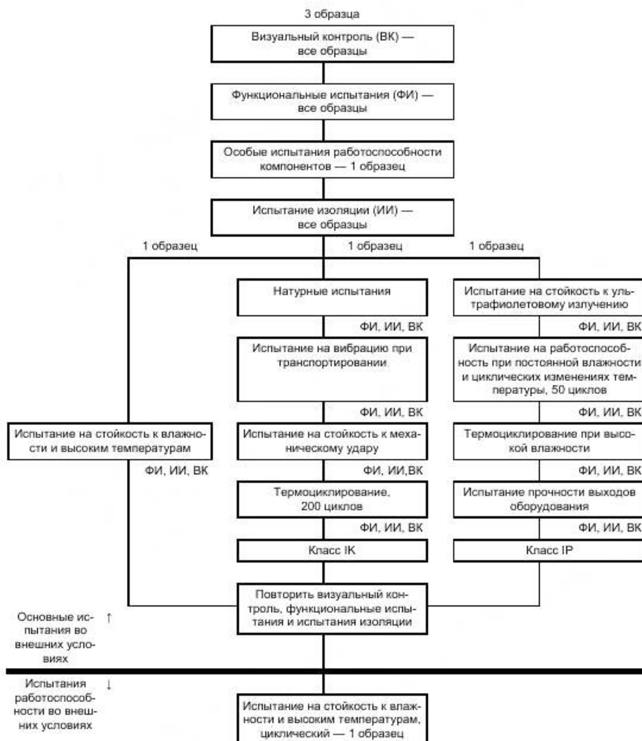
Рисунок 1 — Последовательность испытаний
