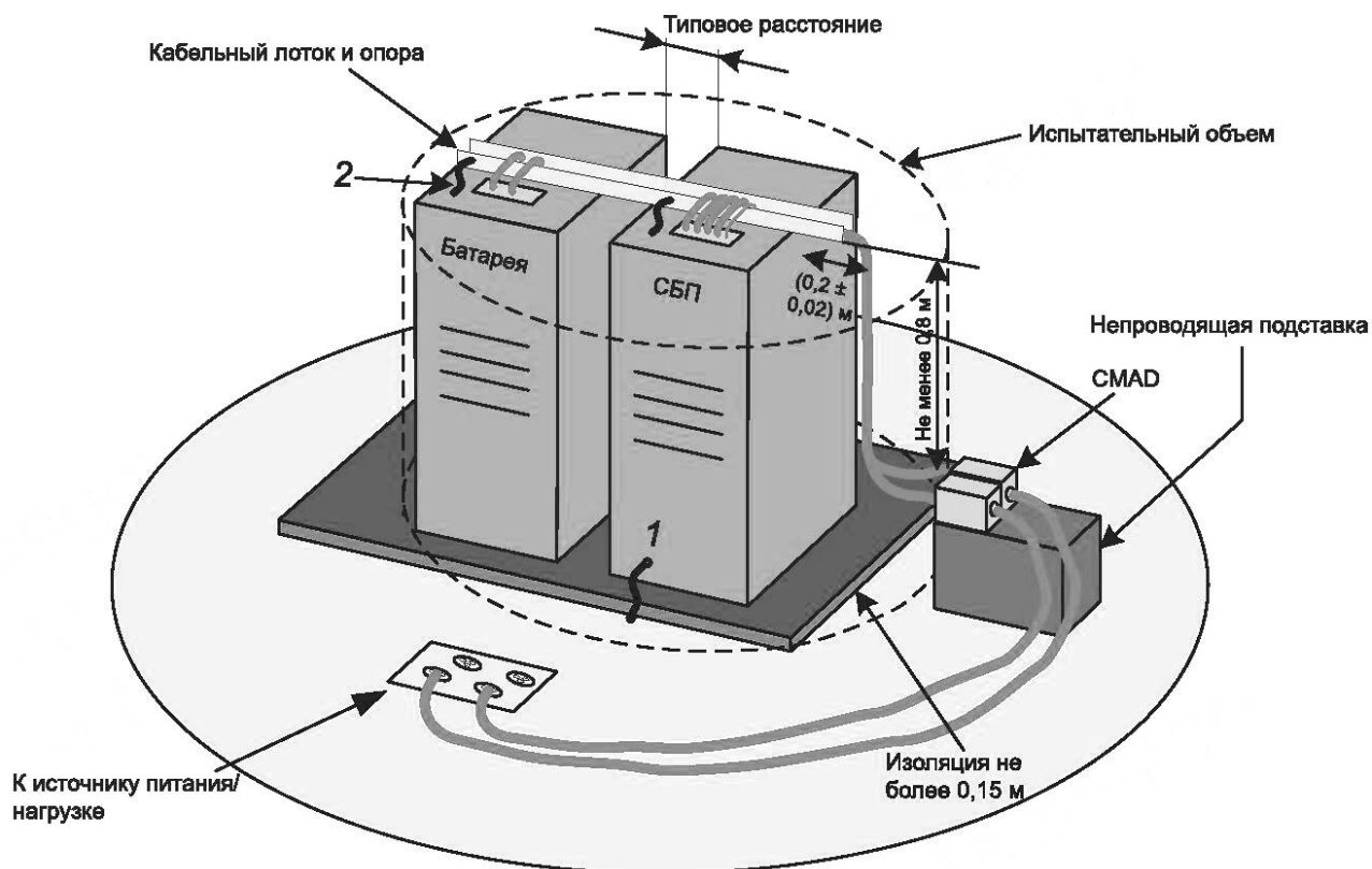
1 — специальная клемма заземления для обеспечения ЭМС (если имеется); 2 — кабельные лотки или каналы, если они проводящие, должны быть заземлены согласно соответствующим правилам электромонтажа
