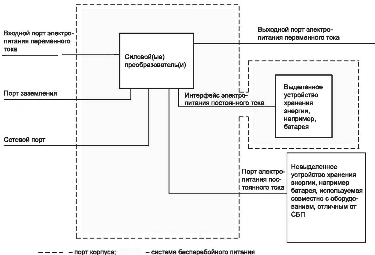
Рисунок 1 — Порты СБП
