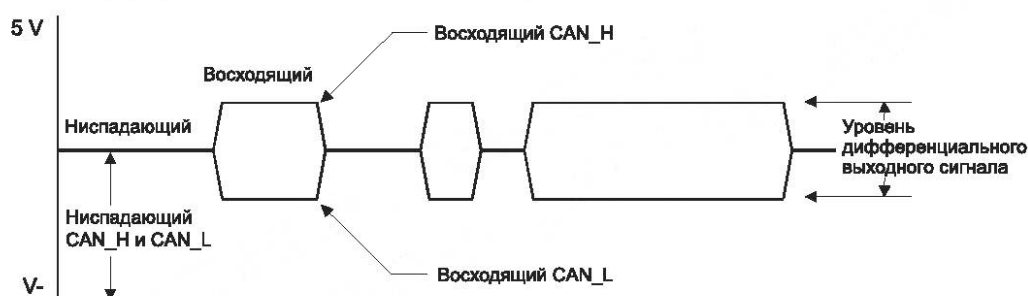
Рисунок 69 — Уровни передачи
