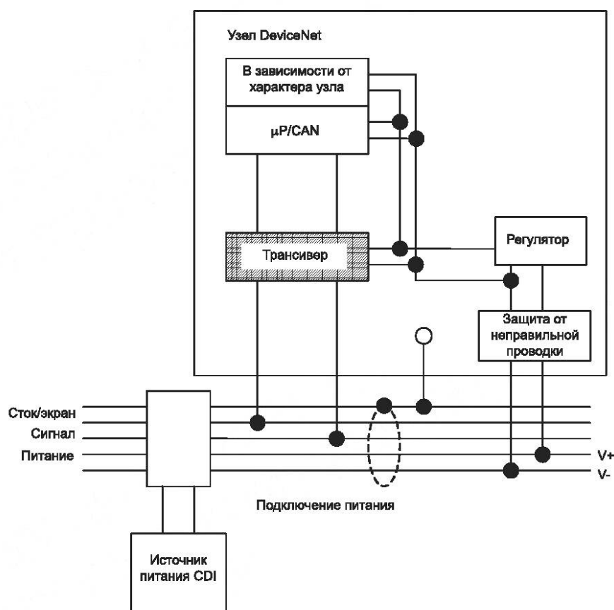
Рисунок 48 — Устройство, содержащее неизолированный физический уровень
