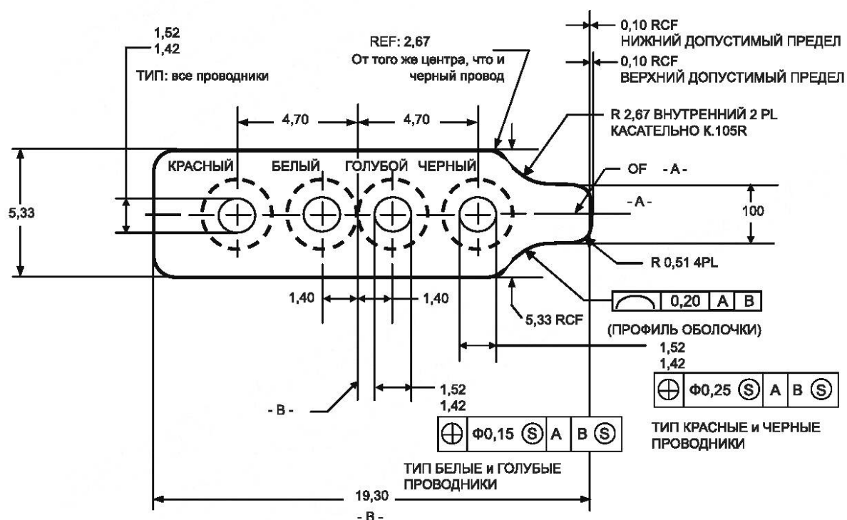
Рисунок 55 — Плоский кабель: физическая конфигурация
