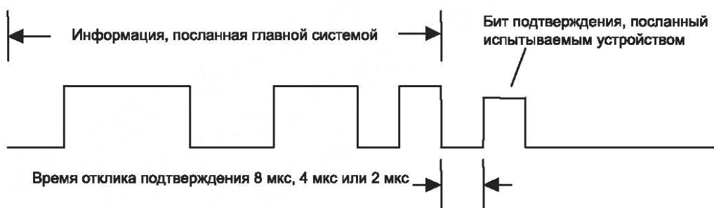
Рисунок 71 — Временная выдержка
