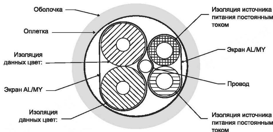
Рисунок 53 — Тонкий кабель: физическая конфигурация
