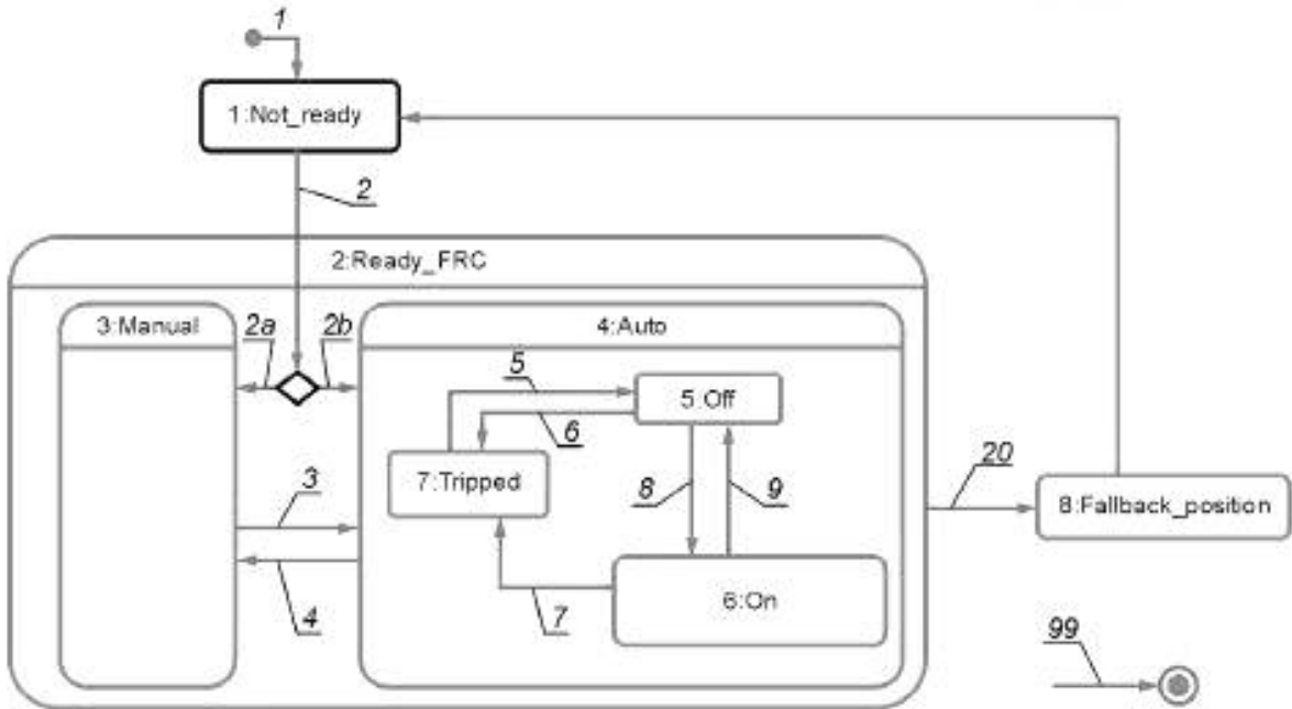
1, 2, 2a, 2b, 3, 4, 5, 6, 7, 8, 9, 20, 21, 99 — переходы состояний пускателя управления двигателем. 1, 2, 3, 4, 5, 6, 7, 8 — состояния пускателя управления двигателем.
