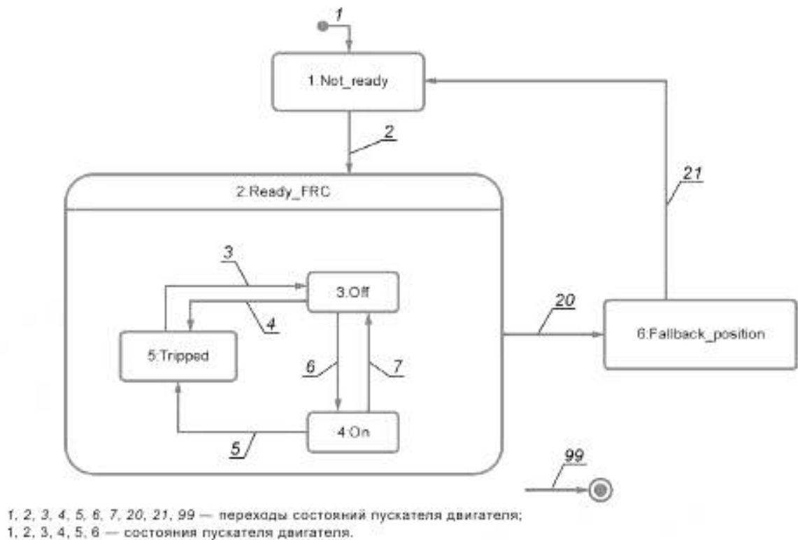
Рисунок 1 — Блок-схема состояний пускателя двигателя
