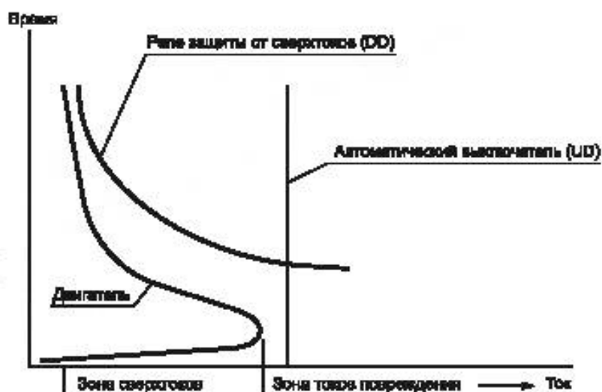
Рисунок 5 — Селективность между автоматическим выключателем мгновенного действия (ABM) и реле защиты от сверхтоков
