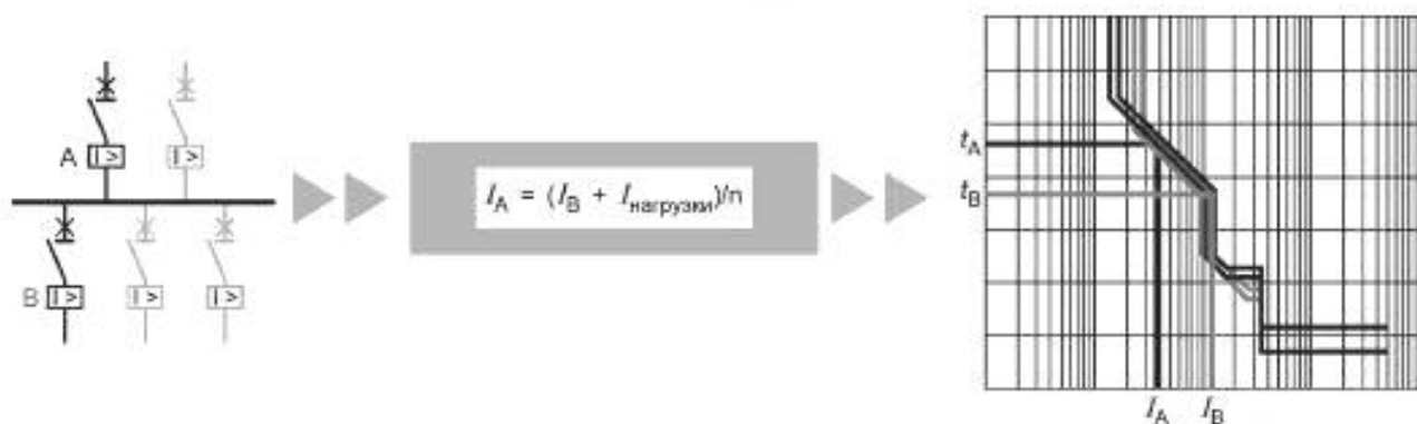
Рисунок В.2b — Последовательно включенные УТЗ (ОСРД), несколько нагрузок (разветвляющийся ток)
