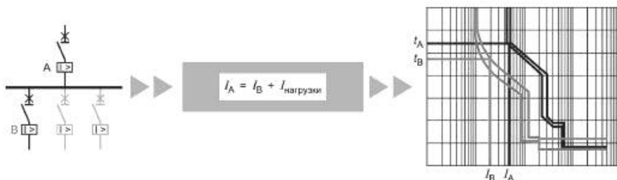
Рисунок В.2b — Последовательно включенные УТЗ (ОСРД), несколько нагрузок (разветвляющийся ток)
