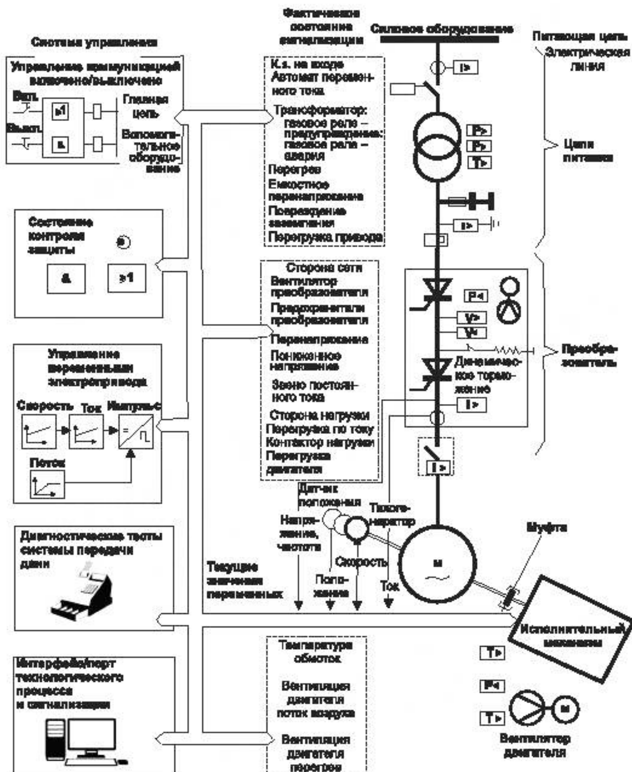
Рисунок 1 – Функциональная схема электропривода переменного тока
