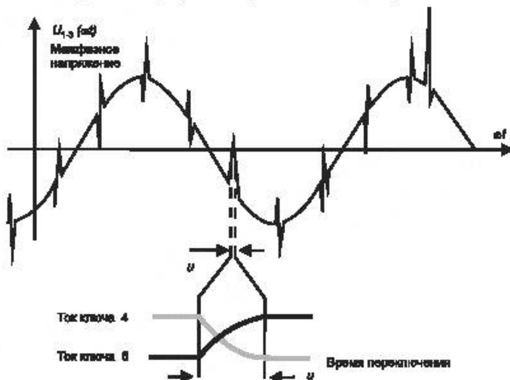
Рисунок В.12 – Трехфазный 6-пульсный мостовой преобразователь
