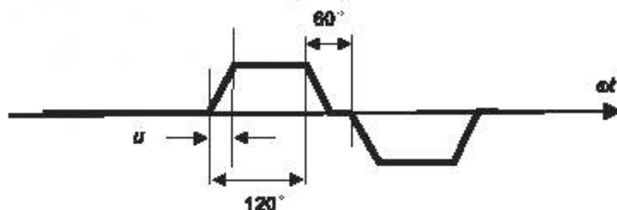
Рисунок В.3 – Трапецевидный ток питания
