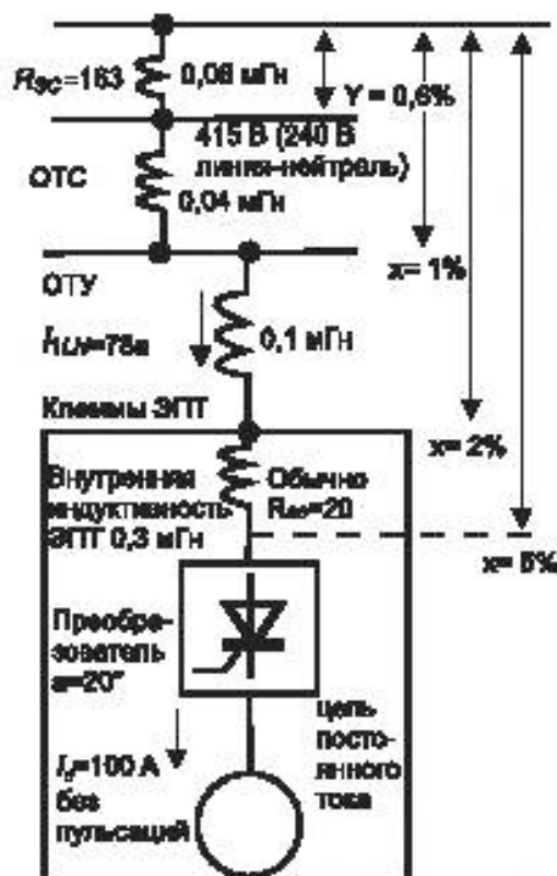
Рисунок В.11 – Пример простой структуры
