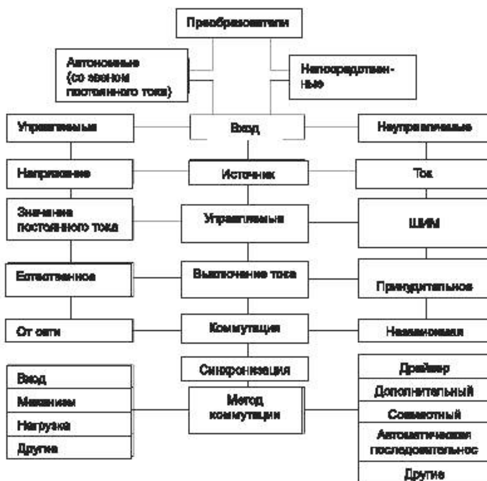
Рисунок F.1 – Конфигурации преобразователей переменного тока
