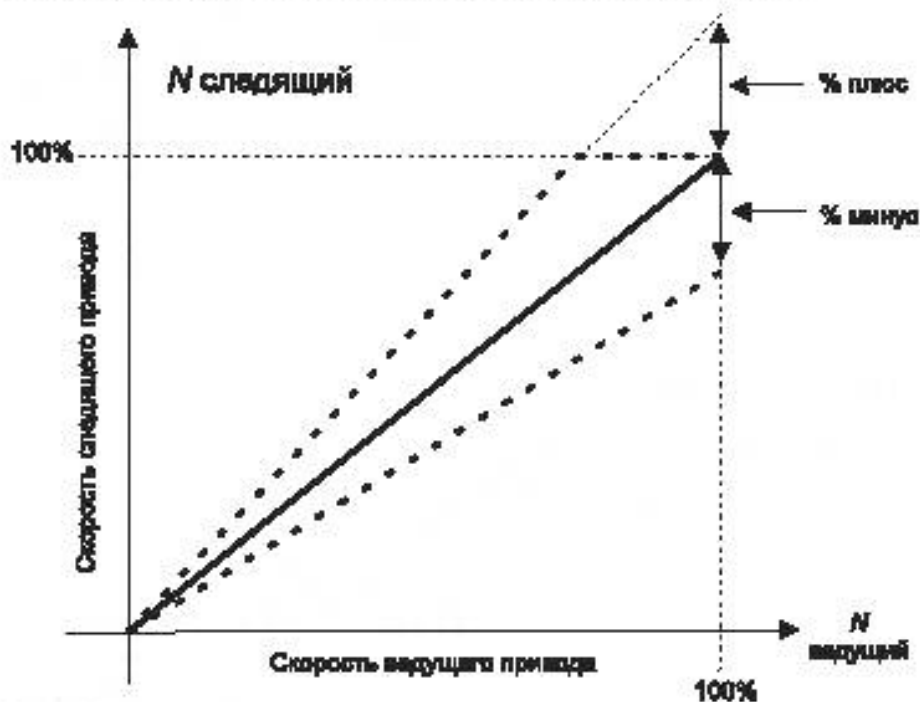
Рисунок D.11 – Пропорциональная зависимость скоростей ведущего/следящего электропривода
