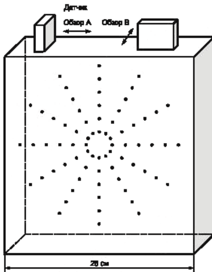
Рисунок A.1 — Решетка нейлоновых нитей в виде концентрических кругов
