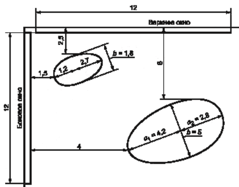
Рисунок В.1 — Фантом с тканеимитирующими яйцеобразными мишенями
