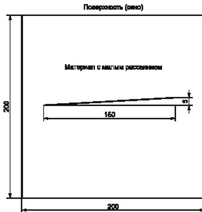
Рисунок С.2 — Тест-объект для оценки осевого разрешения
