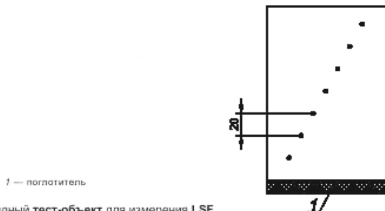
Рисунок С.1 — Нитевидный тест-объект для измерения LSF
