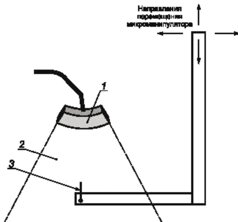
1 — преобразователь; 2 — обзорное поле; 3 — линейная мишень
