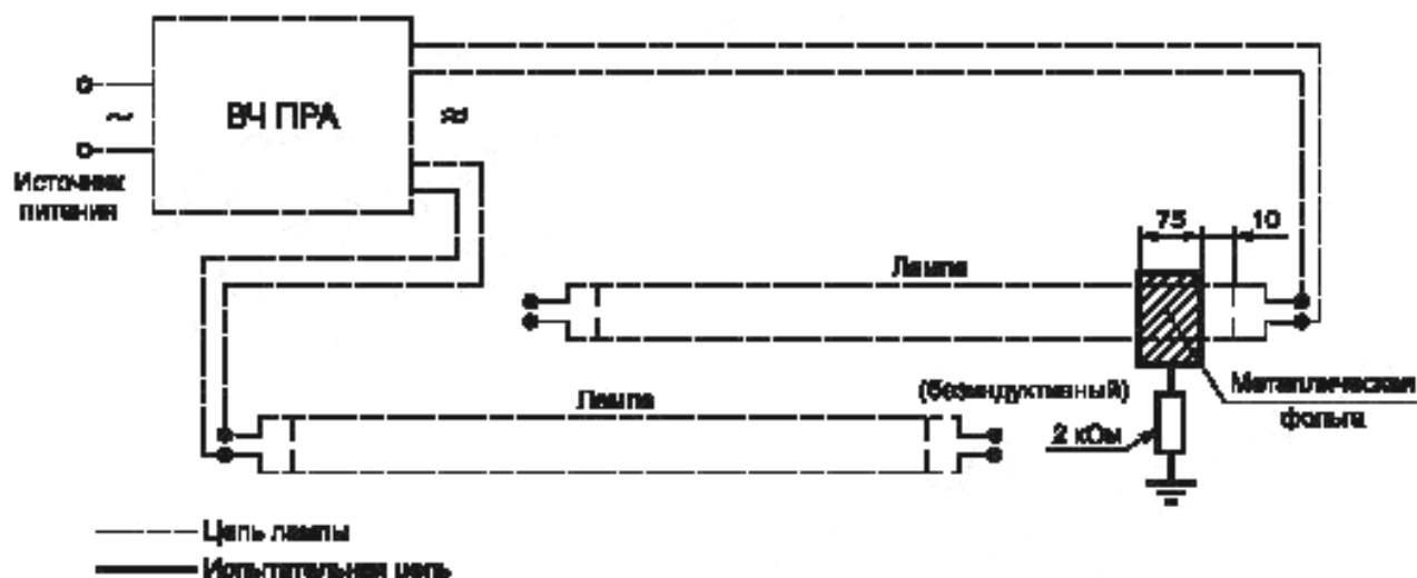
Рисунок I.1 — Испытательная установка
