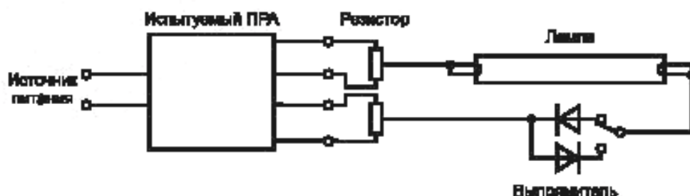
а — Схема испытания
