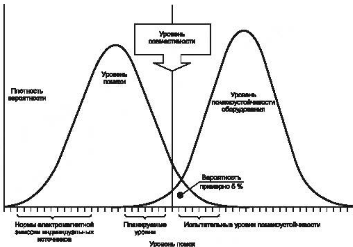
Рисунок А.1 — Уровни электромагнитной эмиссии/помехоустойчивости и уровень совместимости с примером уровней электромагнитной эмиссии/помехоустойчивости для одиночных эмиттера и рецептора как функции некоторых независимых переменных (см. IEC 61000-1-1)
