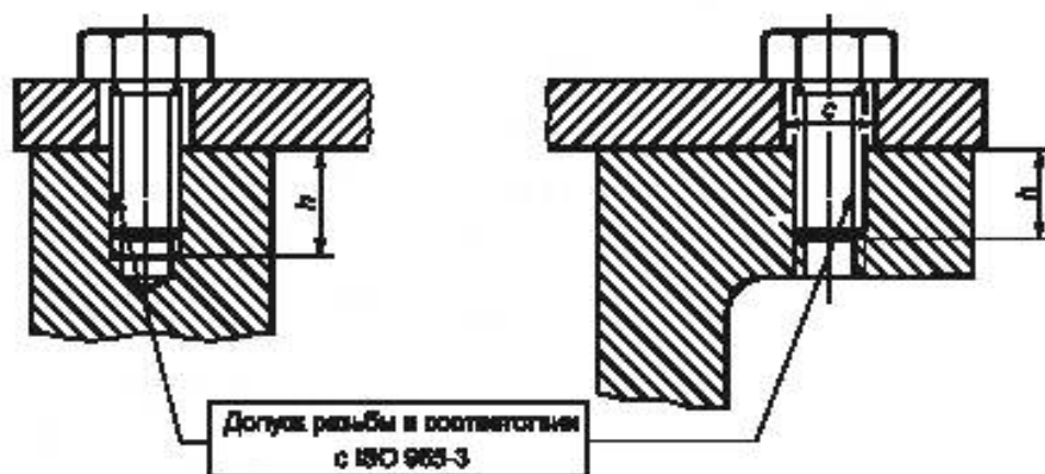
Рисунок 2 — Допуски и зазор для нарезных крепежных деталей
