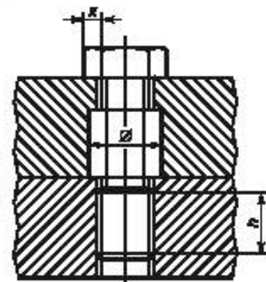
Ø — отверстие со стандартным зазором для прохода резьбы соответствующей формы; h не менее основного диаметра резьбы крепежной детали; X — опорный размер крепежной детали с уменьшенным телом; X не менее опорного размера стандартной головки стандартной крепежной детали (с полным телом) с резьбой используемого размера по всей длине
