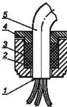
1 — точка разветвления проводников; 2 — уплотнительное кольцо; 3 — тепло кабельного ввода; 4 — зажимное кольцо с изогнутой кромкой; 5 — кабель
