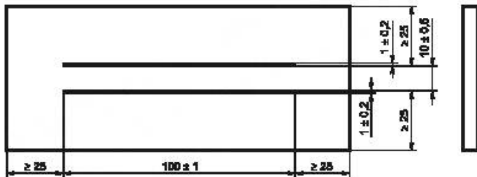
Рисунок 4 — Испытательный образец с электродами из проводящей краски
