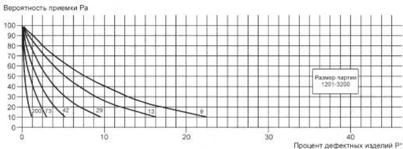
Рисунок С.9 — Объем партии от 501 до 1200
