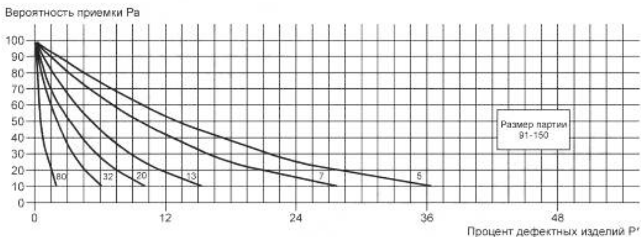
Рисунок С.5 — Объем партии от 51 до 90
