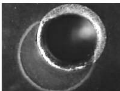
Попадание паяльной маски на монтажную контактную площадку
