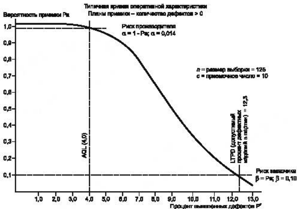
Рисунок 1 — Типичная кривая оперативных характеристик для плана c \geq 0
