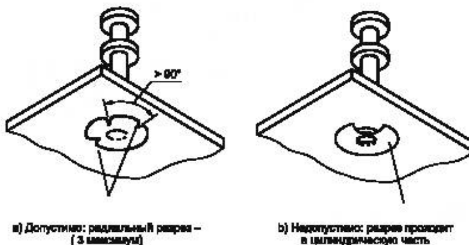
Рисунок 2 — Разрывы развальцованного фланца, обжатого руликом
