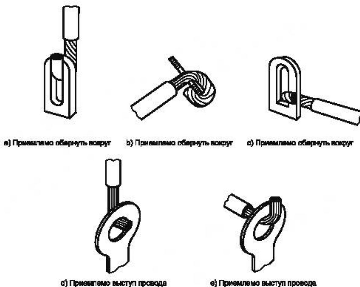
Рисунок 12 — Намотка провода на перфорированный контакт
