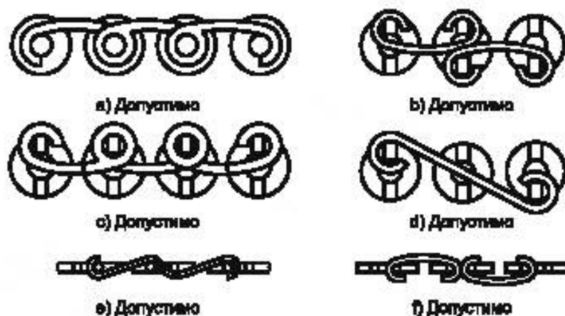
Рисунок 8 — Закрепление провода в последовательный ряд
