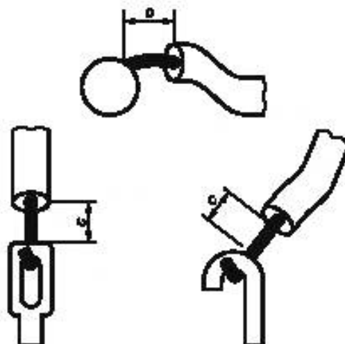
Рисунок 10 — Измерение изоляционного зазора (с)
