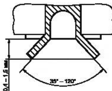
Рисунок 4 — Углы развальцовки фланца
