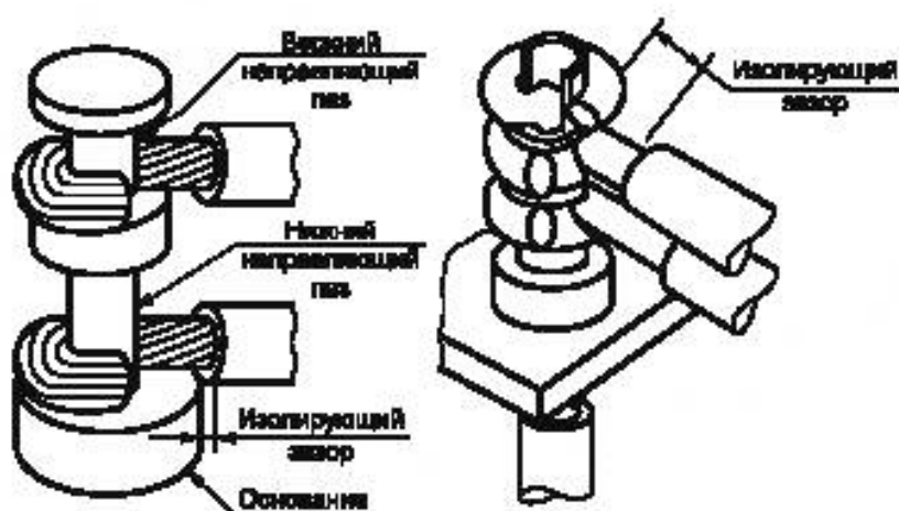
Рисунок 5 — Закрепление проводов или выводов на контактах
