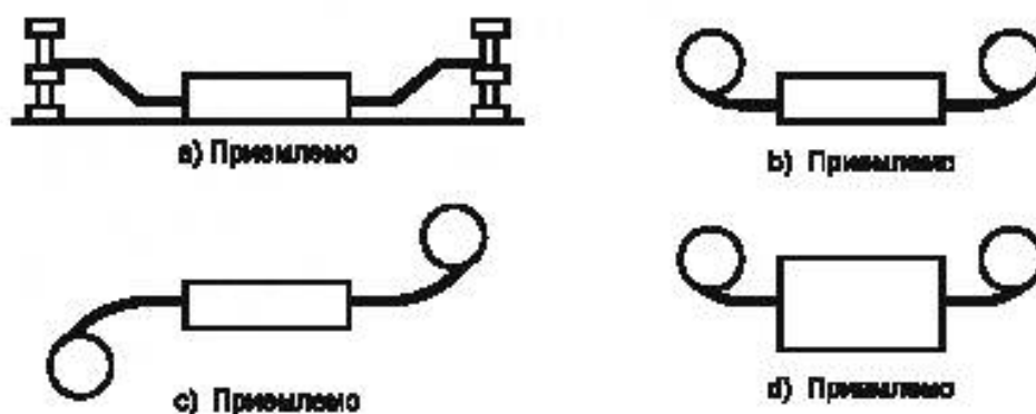
Рисунок 11 — Примеры амортизирующих профилей выводов
