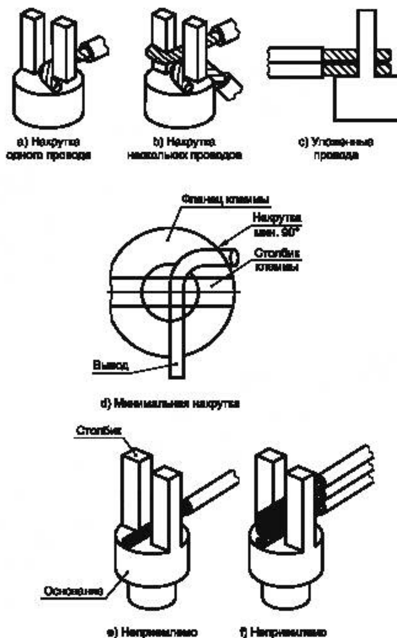
Рисунок 6 — Монтаж в разрезной контакт
