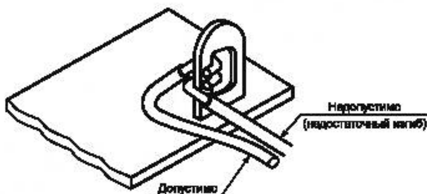
Рисунок 9 — Ремонтнопригодная петля провода
