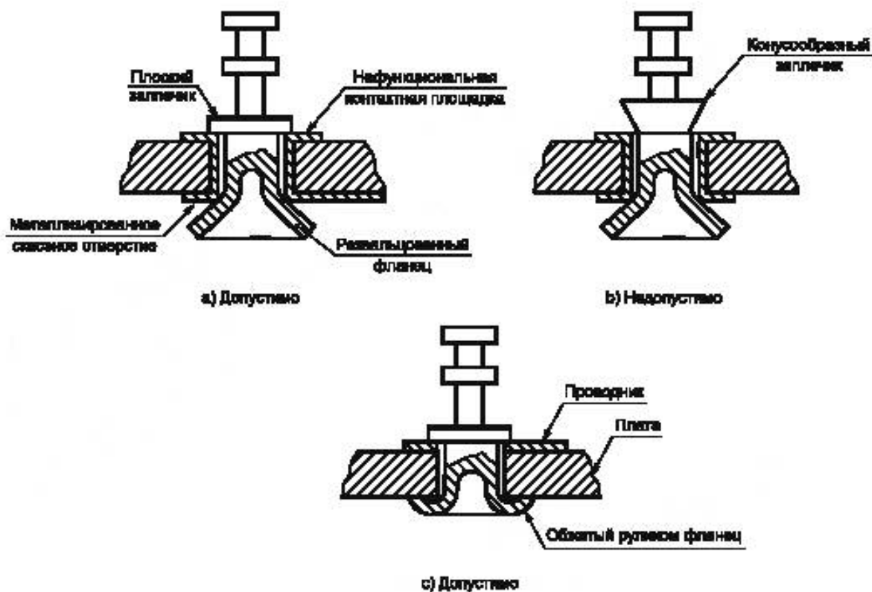
Рисунок 3 — Развальцованные фланцы контакта
