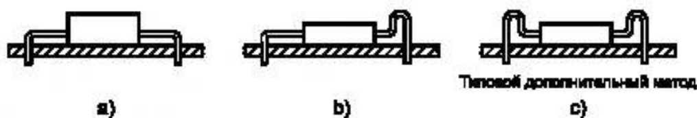
Рисунок А.8 — Примеры формы выводов
