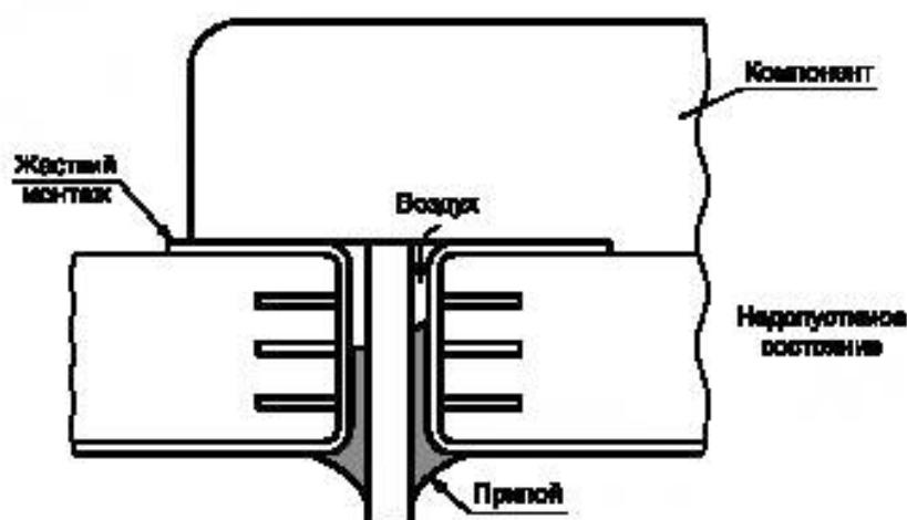
Рисунок 2 — Непропай отверстия
