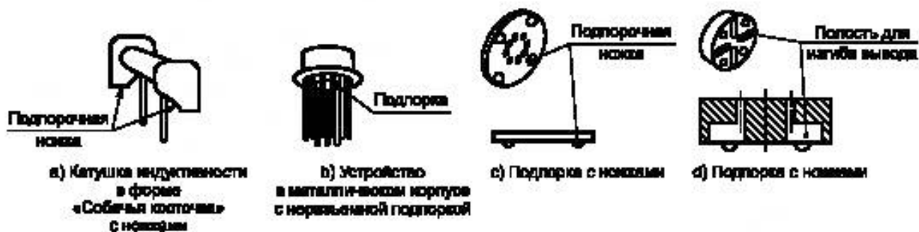
Рисунок А.6 — Монтаж с упорами и подпорками
