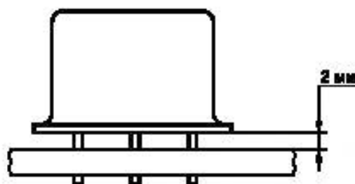
Рисунок А.1 — Монтаж свободно стоящих компонентов
