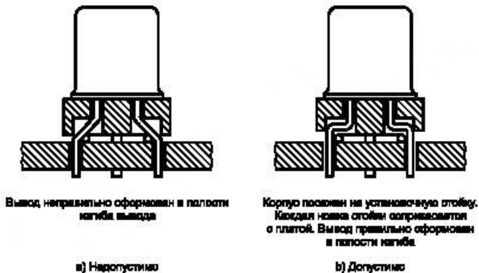
Рисунок А.7 — Неупругие установочные панельки
