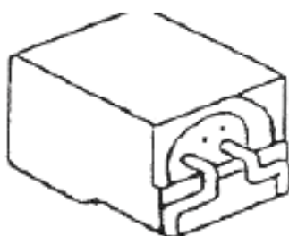
Рисунок 22 – Конструкция безвыводного алюминиевого электролитического конденсатора (горизонтальное исполнение)
